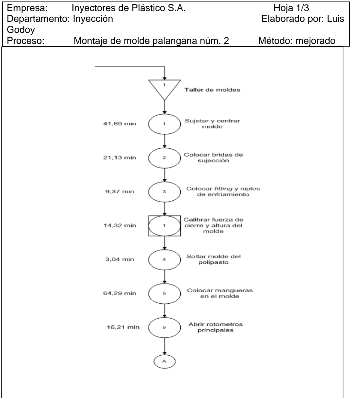
Figura 30. Diagrama de flujo del montaje de molde línea doméstica
