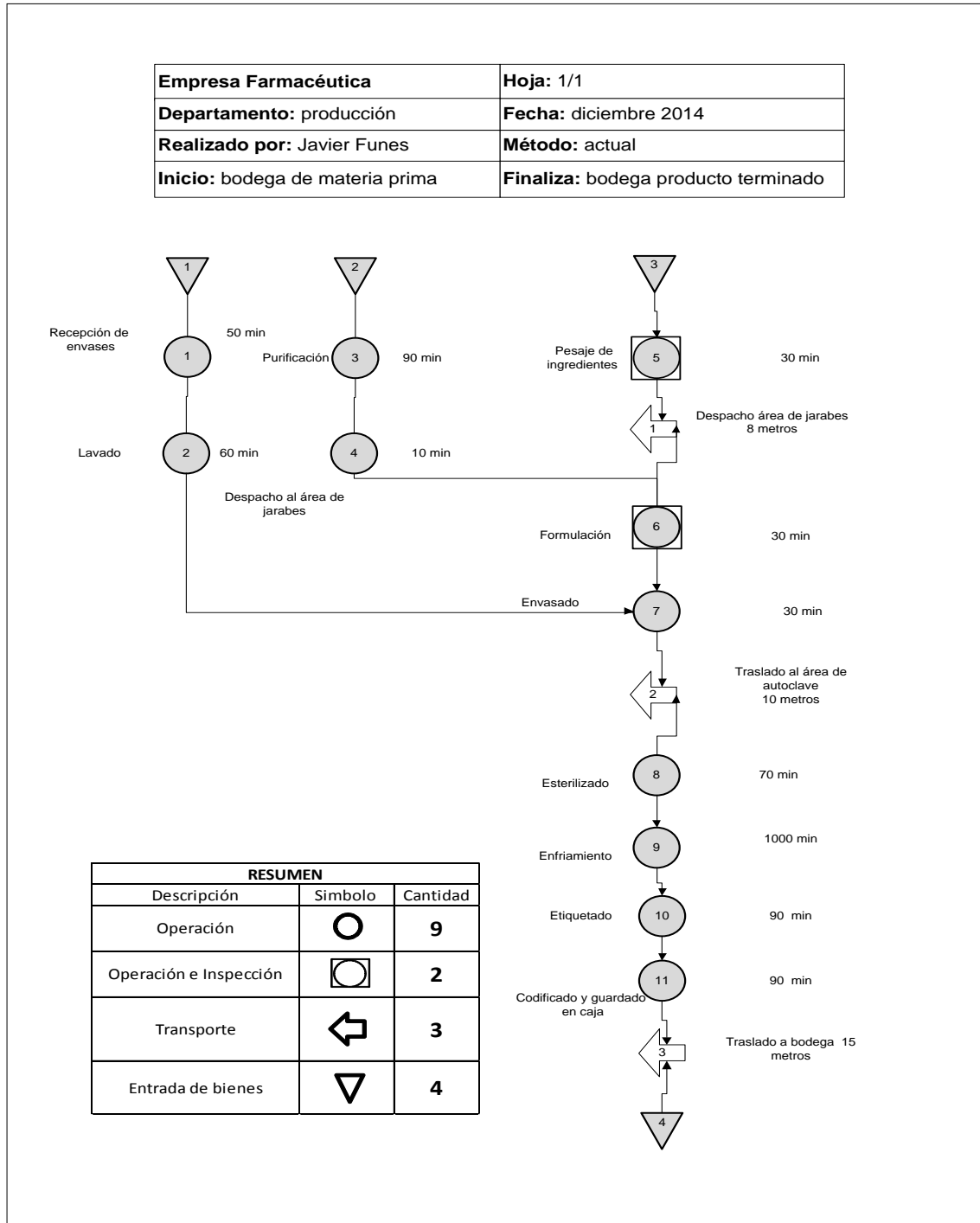
Figura 6. Diagrama del proceso productivo
