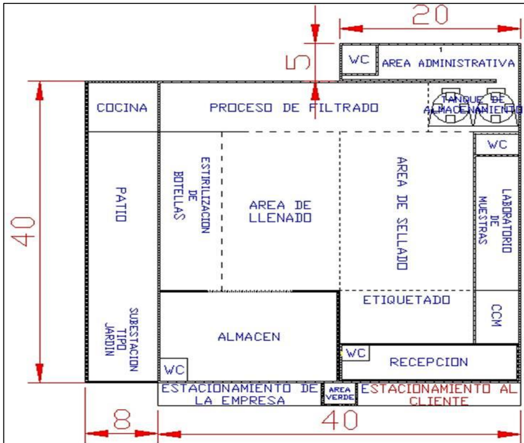
Figura 22. Distribución de planta, producción de suero oral
