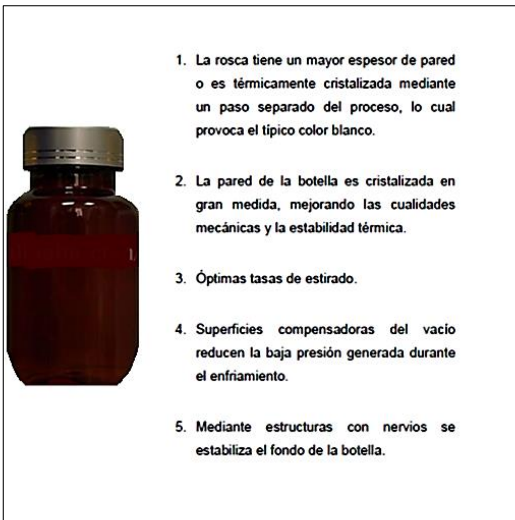
Figura 46. Envase PET para llenado en caliente
