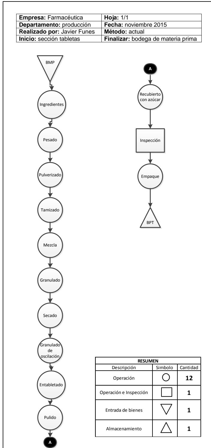
Figura 49. Puntos críticos, sección tabletas
