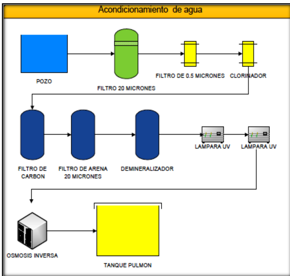
Figura 12. Acondicionamiento del agua
