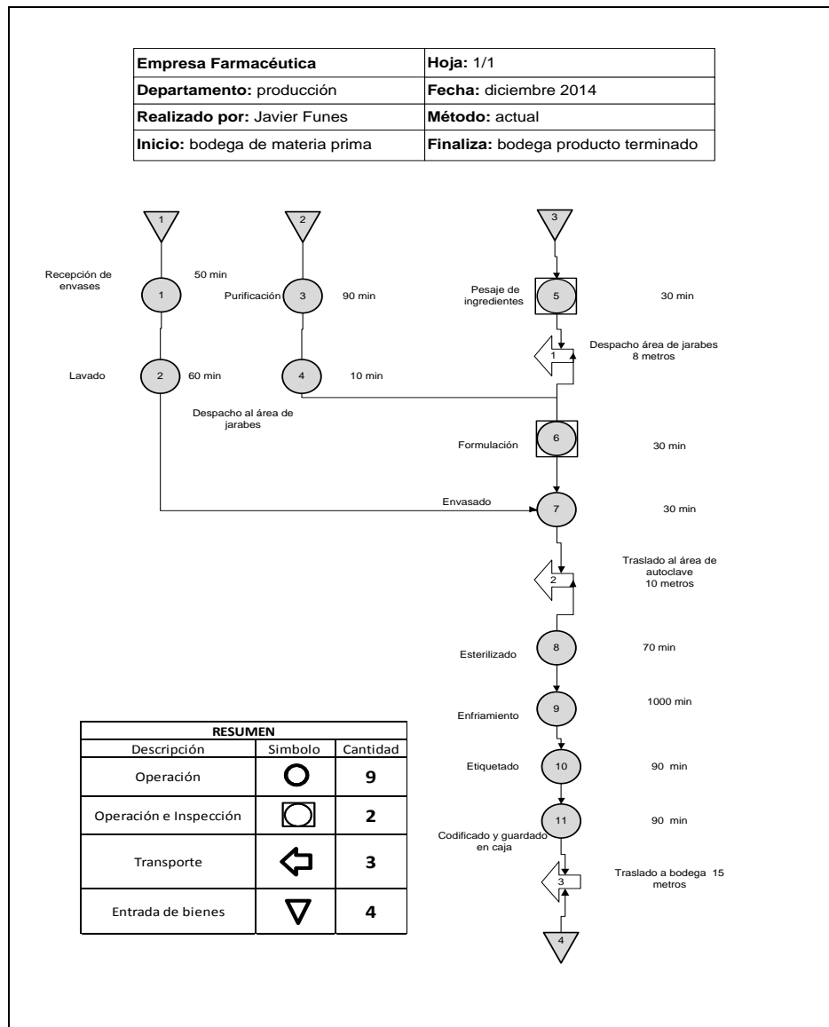
Figura 23. Diagrama de operaciones del proceso
