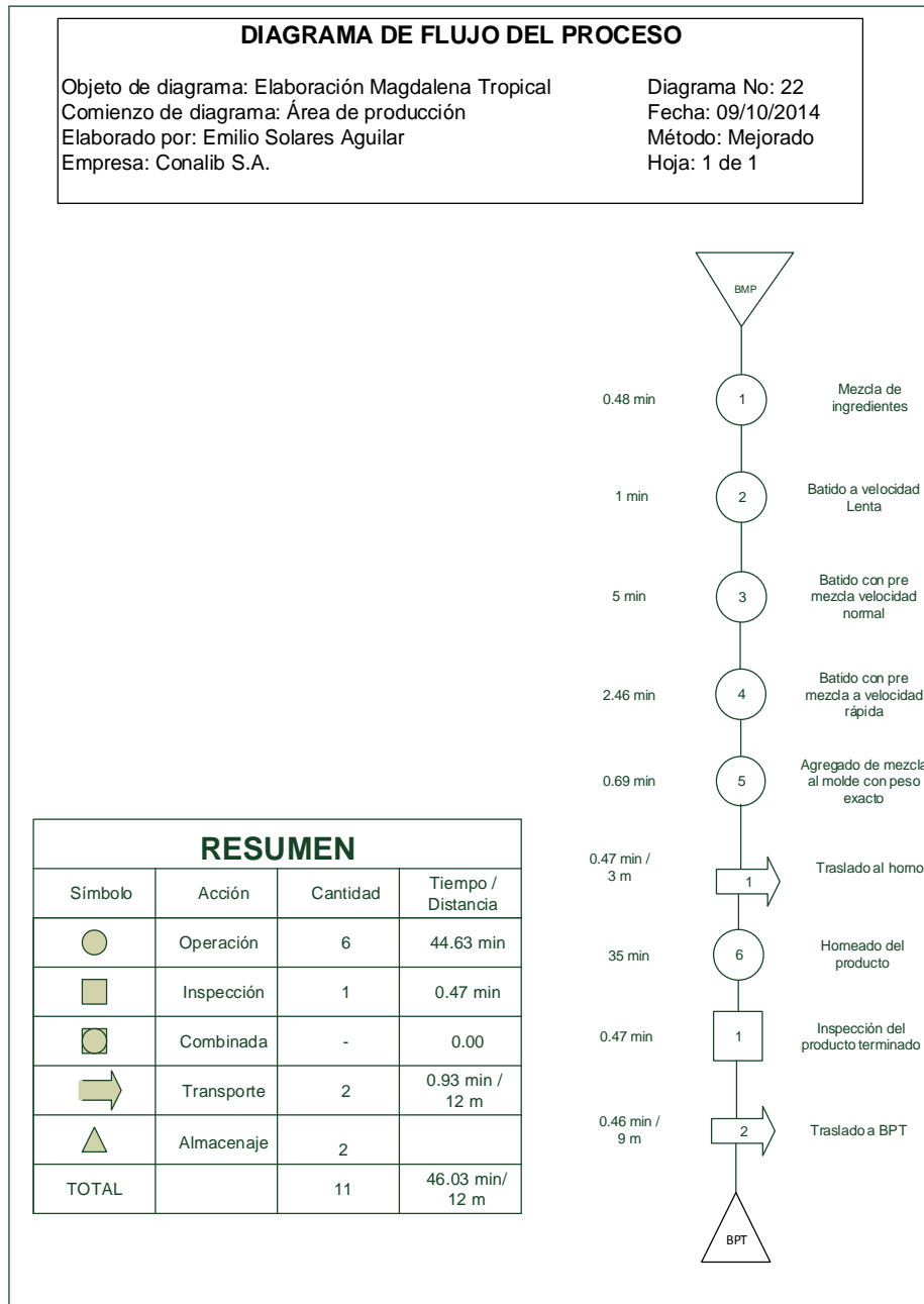
Figura 102. Diagrama de flujo mejorado para la elaboración magdalena tropical
