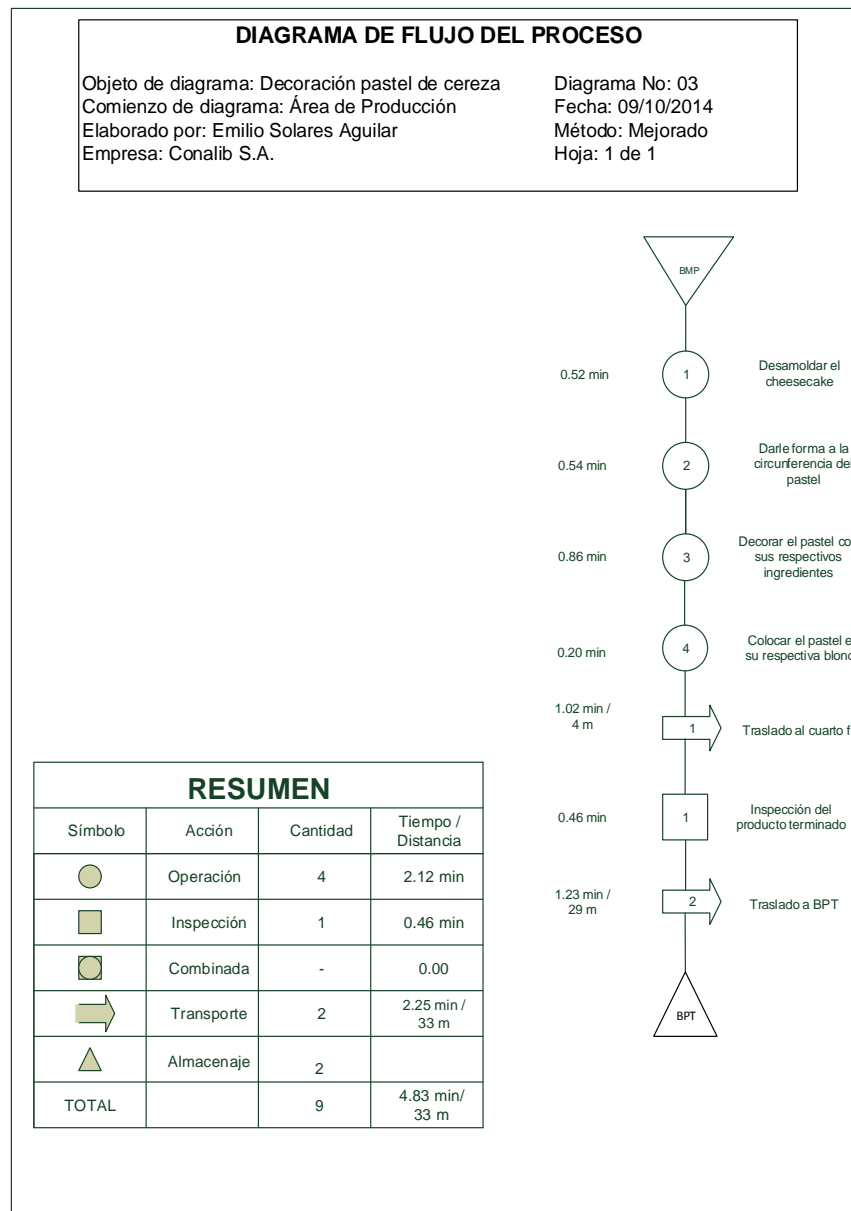
Figura 41. Diagrama de flujo mejorado para la decoración de pastel de cereza
