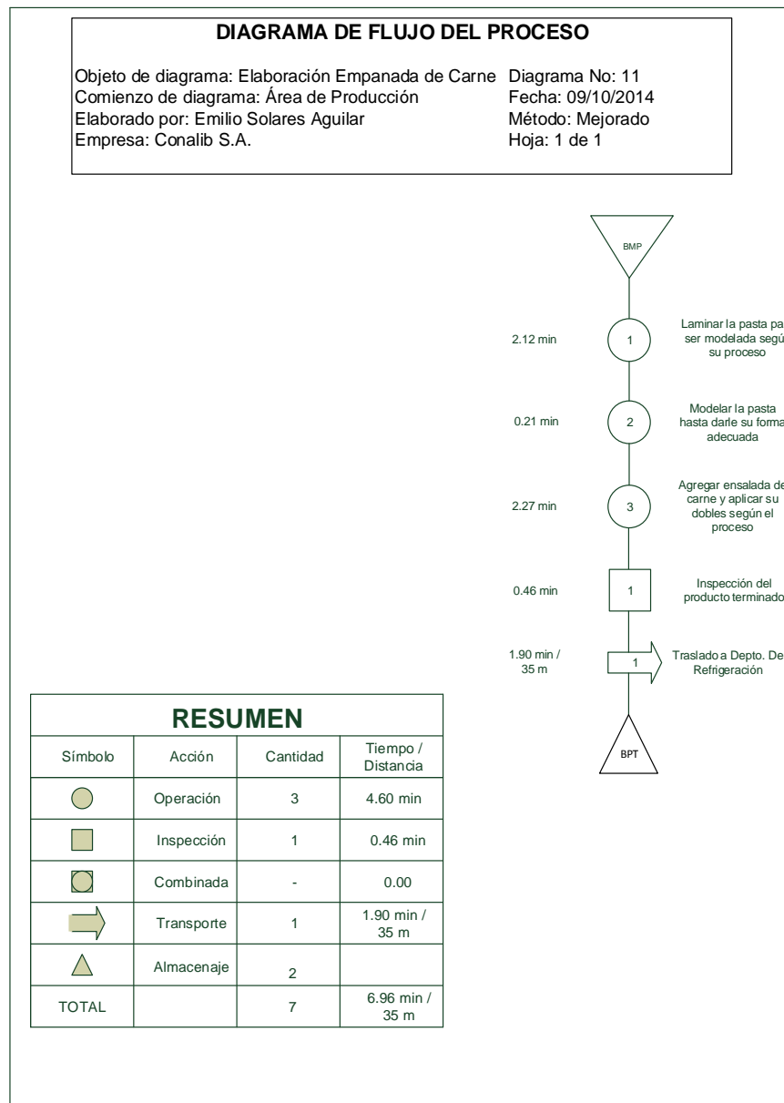
Figura 67. Diagrama de flujo mejorado para la elaboración de empanada de carne
