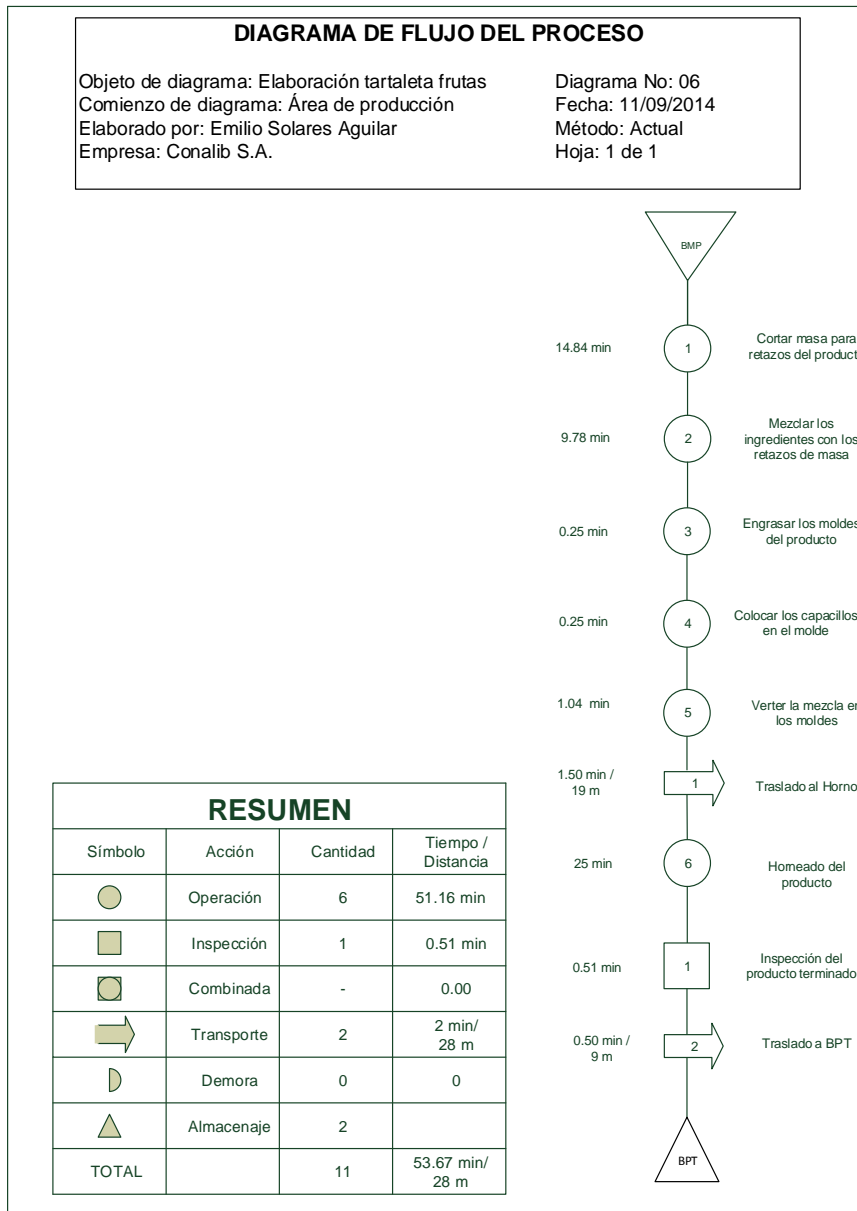
Figura 9. Diagrama de flujo actual de la elaboración de tartaleta de frutas
