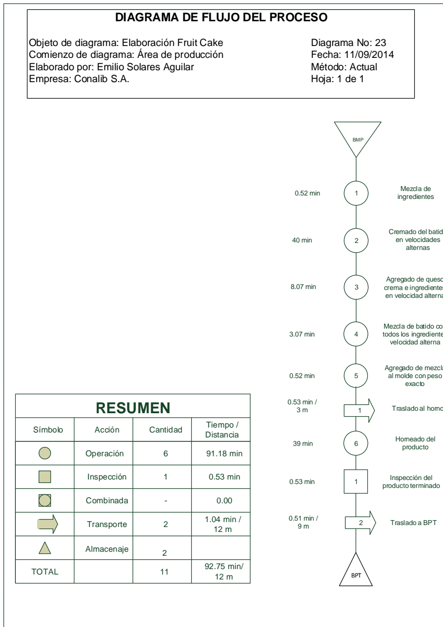
Figura 32. Diagrama de flujo actual de la elaboración de fruitcake
