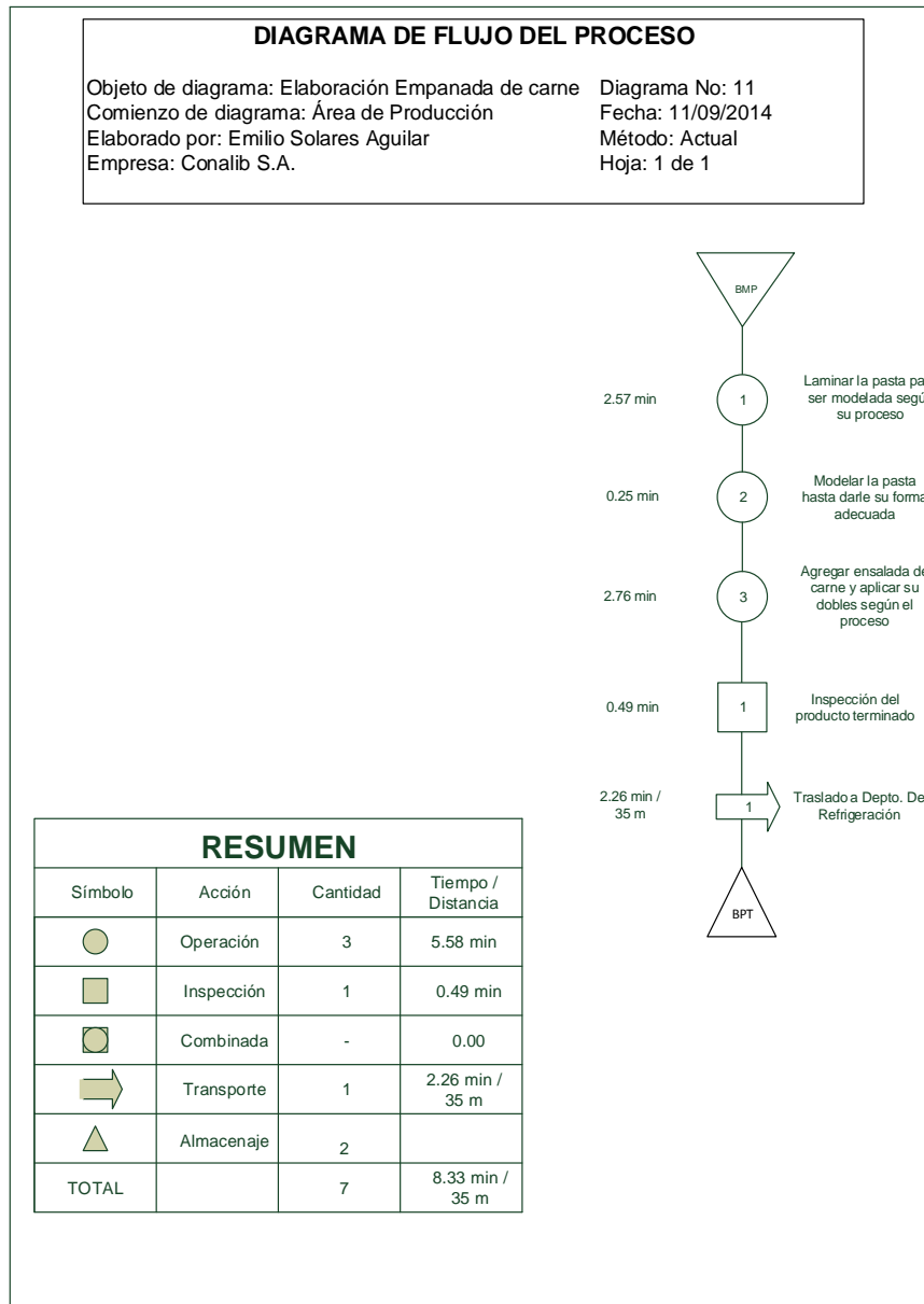
Figura 16. Diagrama de flujo actual de la elaboración de empanada de carne
