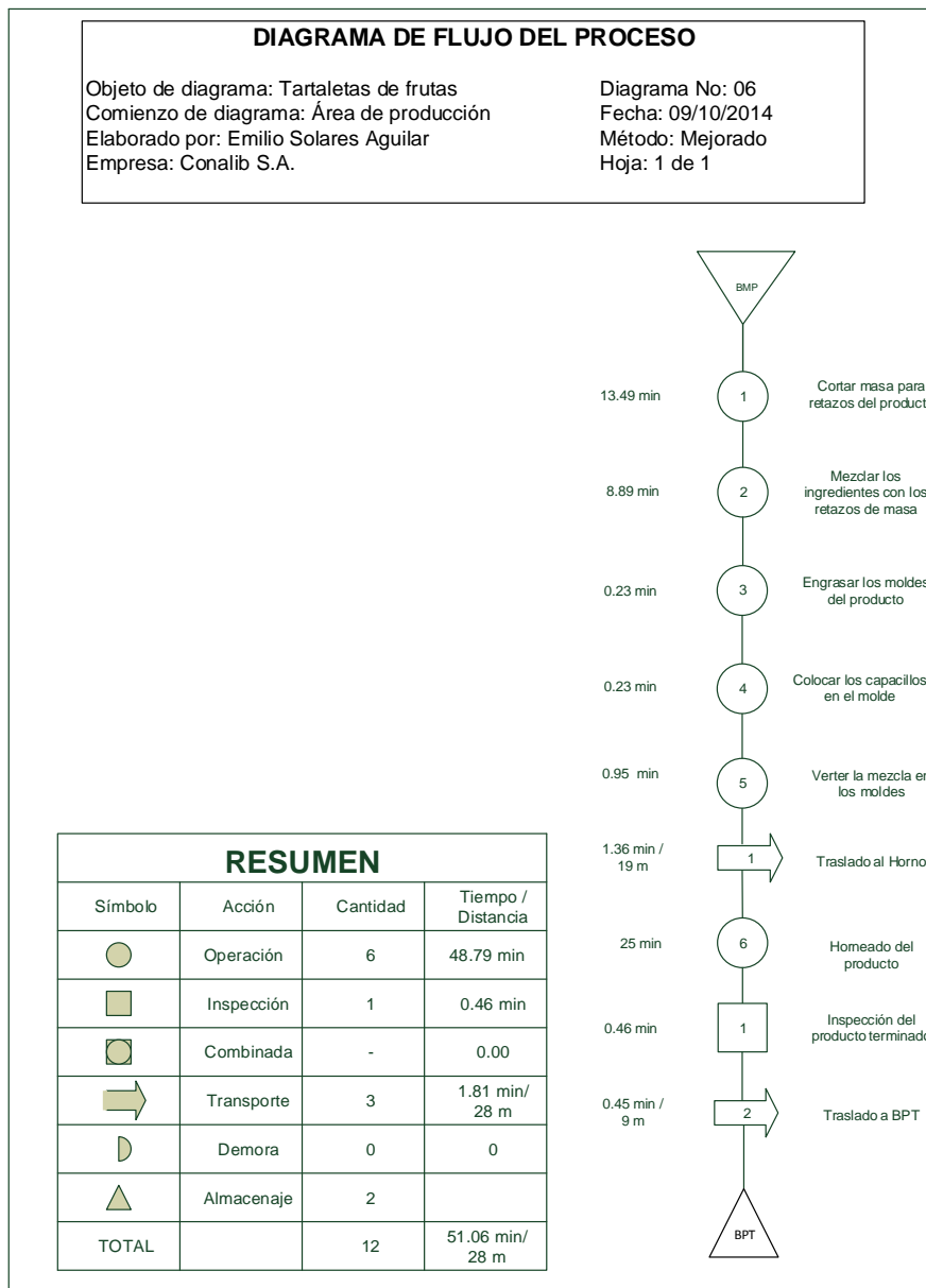
Figura 50. Diagrama de flujo mejorado para la elaboración de tartaleta de frutas
