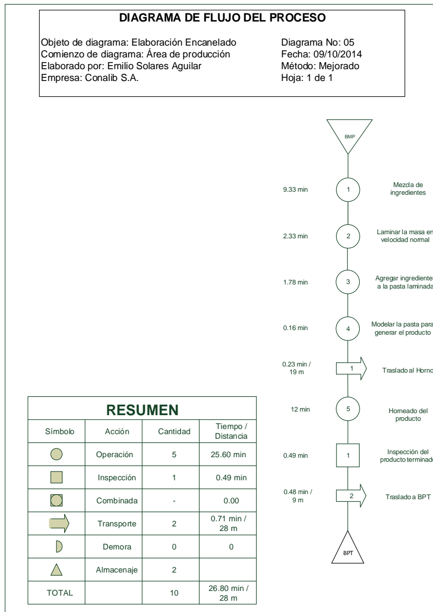
Figura 49. Diagrama de flujo mejorado para la elaboración de encanelado
