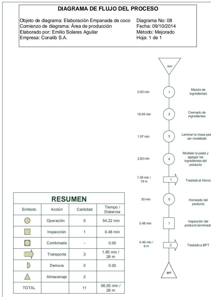
Figura 58. Diagrama de flujo mejorado para la elaboración de empanada de coco
