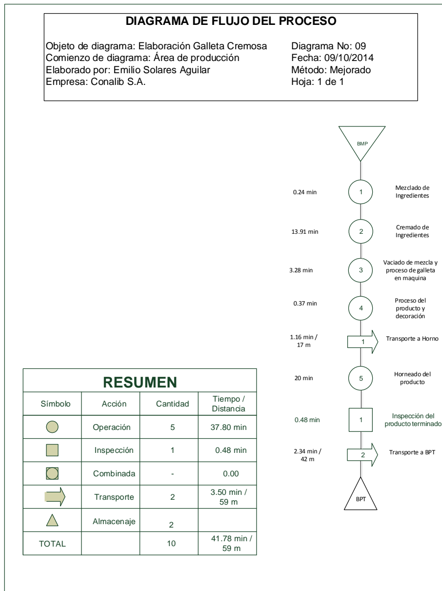
Figura 59. Diagrama de flujo mejorado para la elaboración de galleta cremosa
