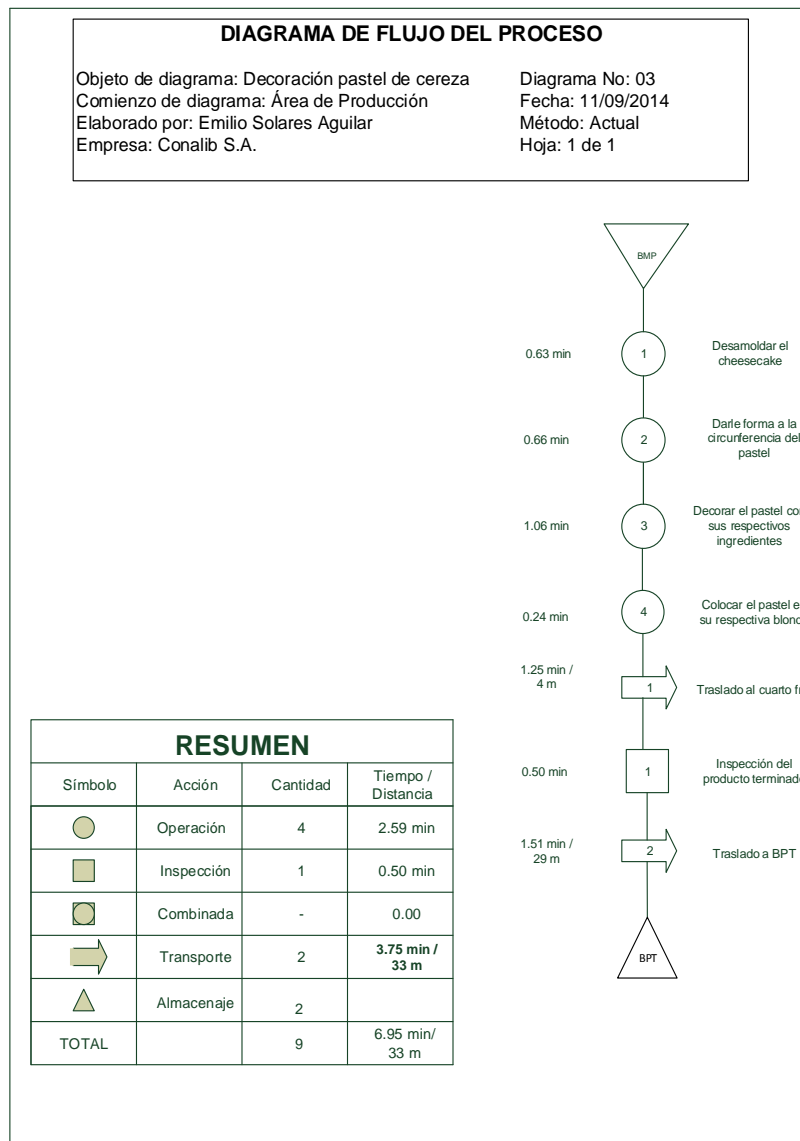
Figura 5. Diagrama de flujo actual de la decoración del pastel de cereza
