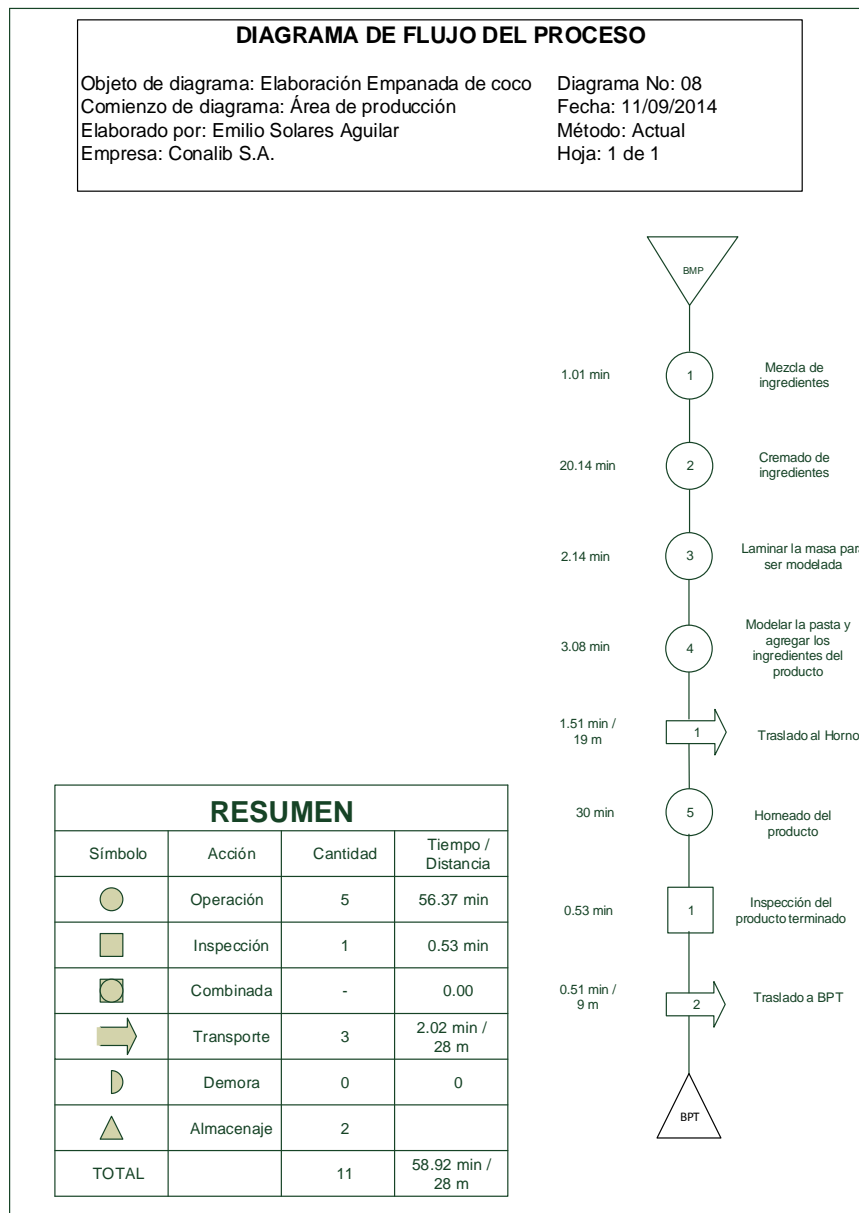
Figura 12. Diagrama de flujo actual de la elaboración de empanada de coco
