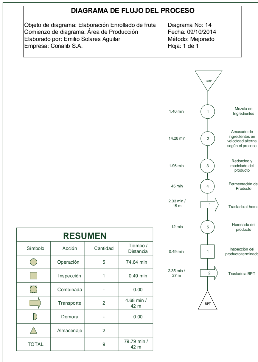
Figura 76. Diagrama de flujo mejorado para la elaboración de enrollado de fruta
