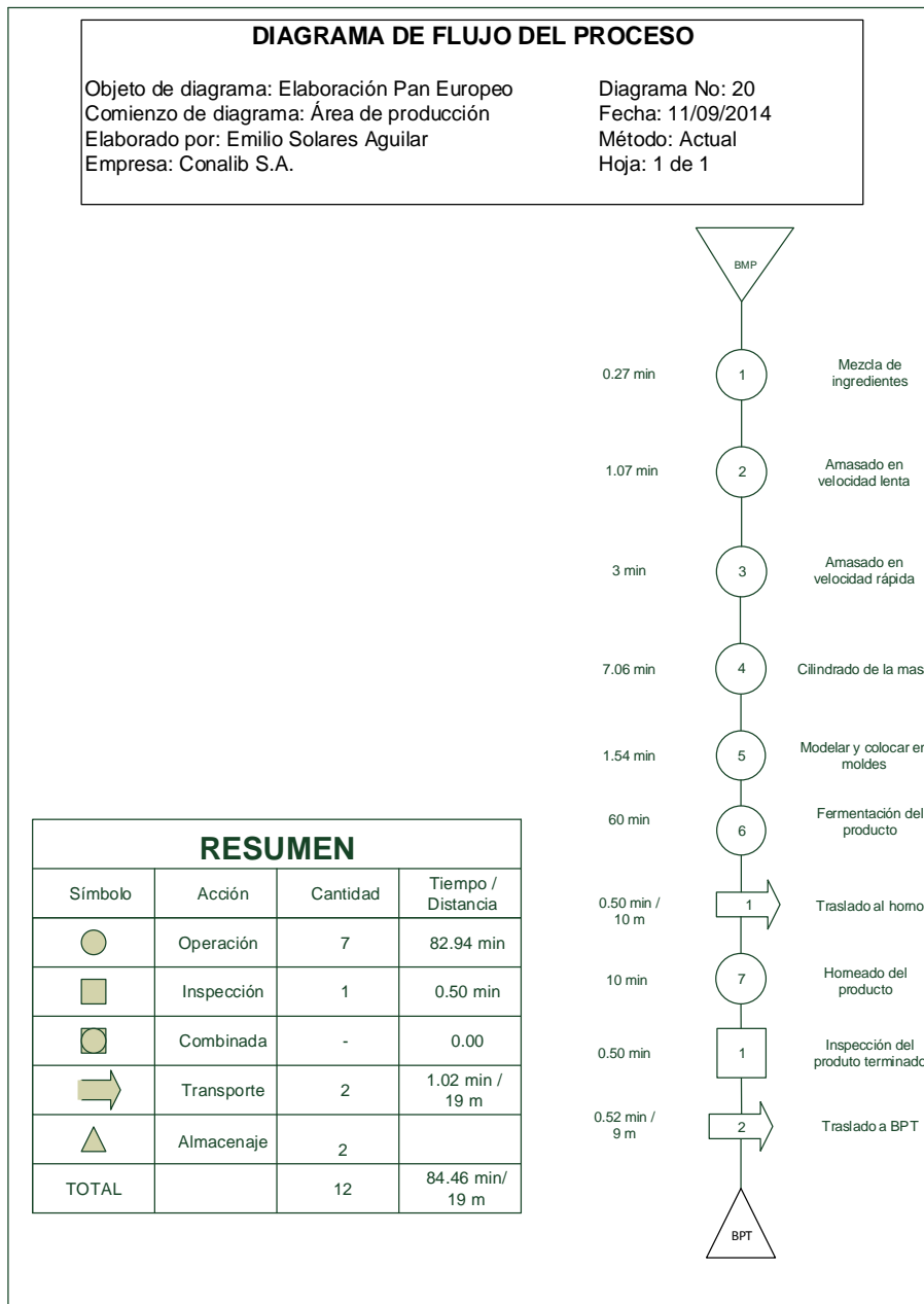
Figura 28. Diagrama de flujo actual de la elaboración de pan europeo
