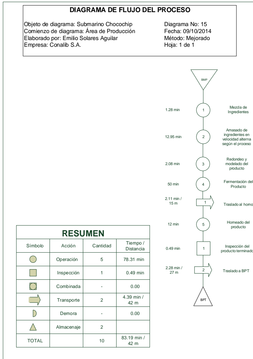
Figura 77. Diagrama de flujo mejorado para la elaboración de submarino chocochip
