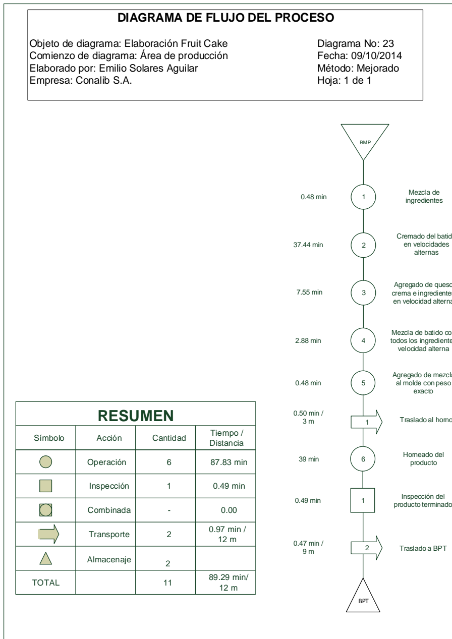
Figura 103. Diagrama de flujo mejorado para la elaboración fruitcake
