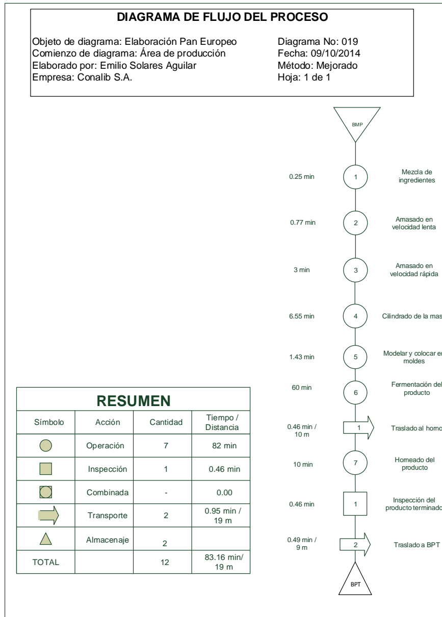
Figura 94. Diagrama de flujo mejorado para la elaboración de pan europeo
