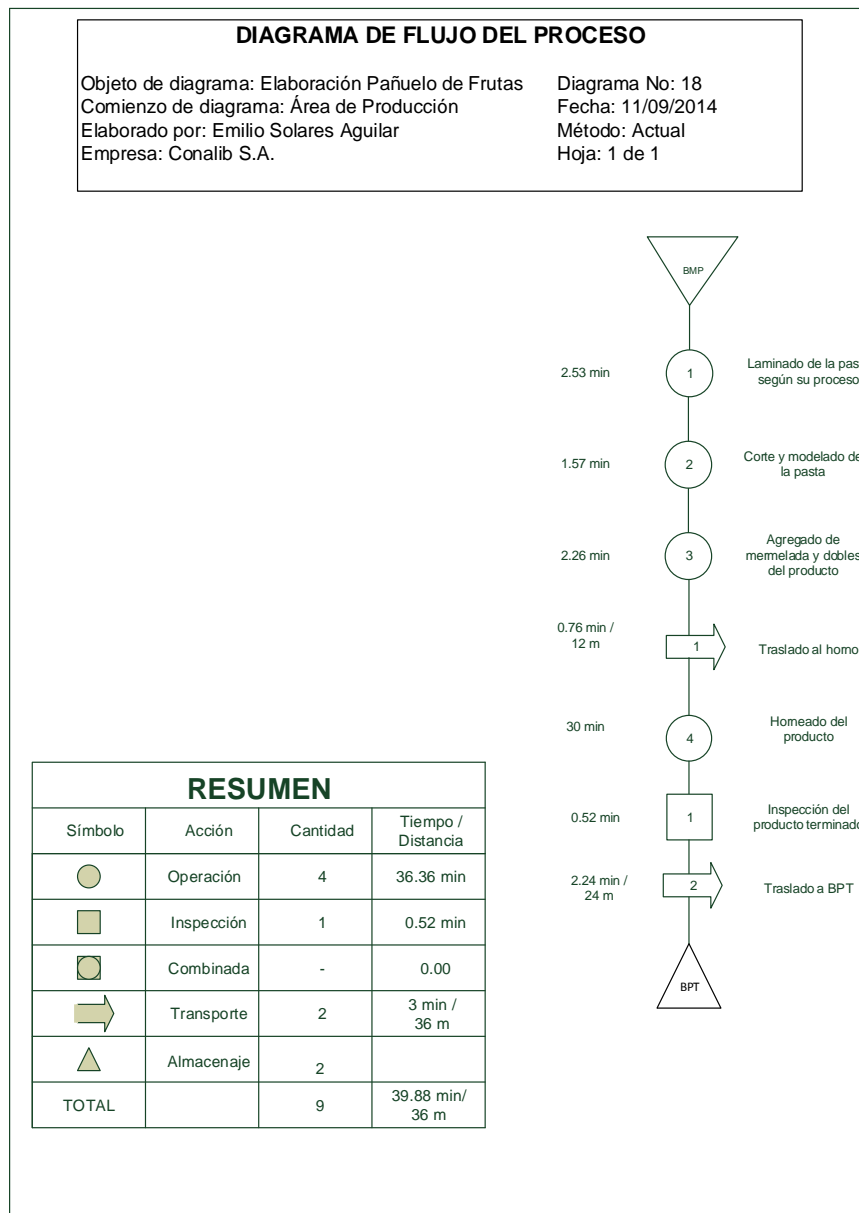
Figura 25. Diagrama de flujo actual de la elaboración de pañuelo de frutas
