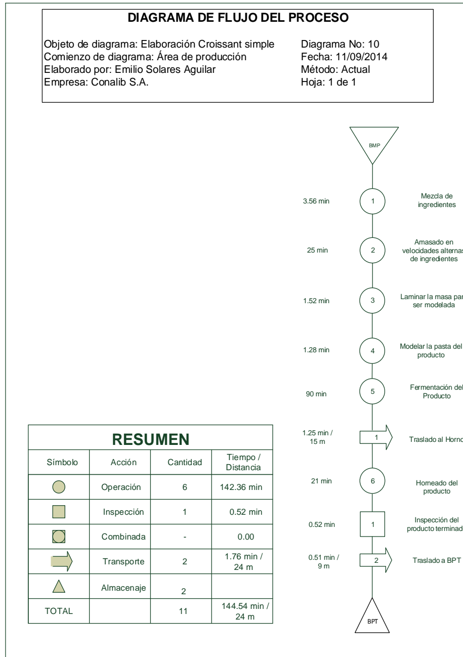
Figura 15. Diagrama de flujo actual de la elaboración de croissant simple
