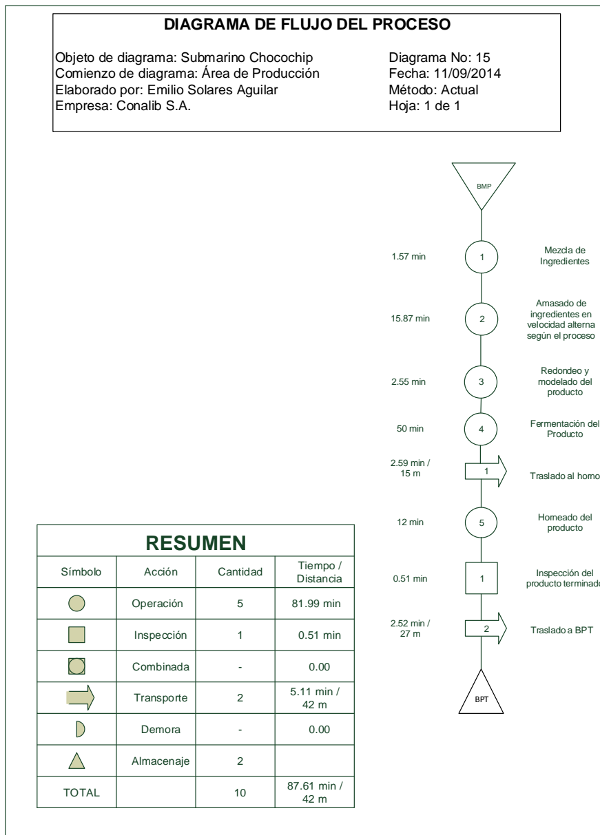
Figura 21. Diagrama de flujo actual de la elaboración de submarino chocochip
