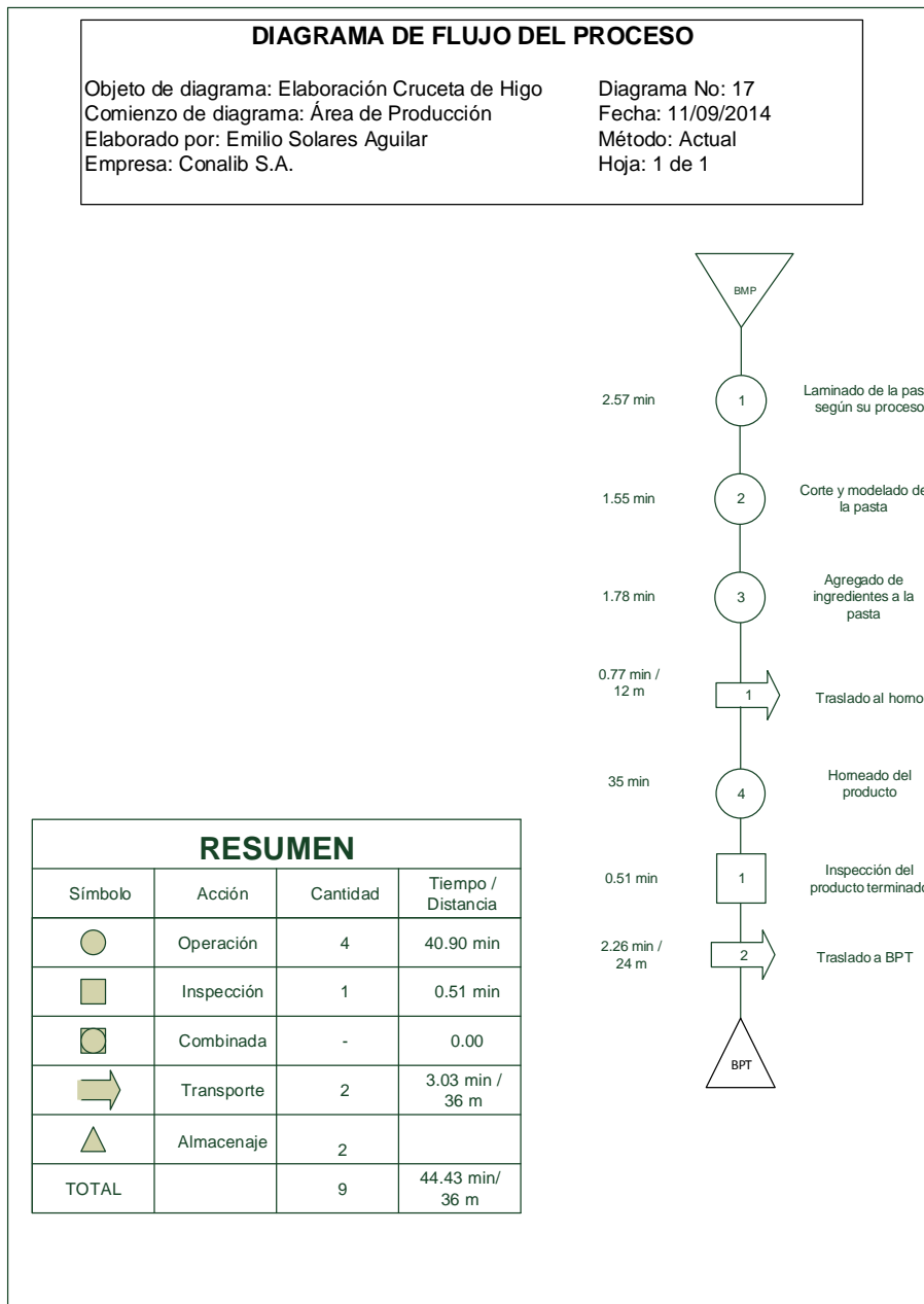
Figura 24. Diagrama de flujo actual de la elaboración de cruceta de higo
