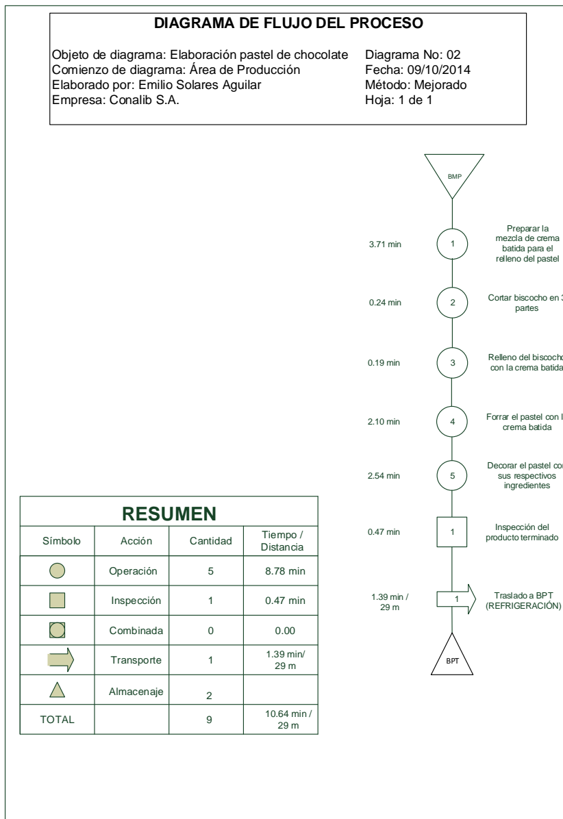
Figura 40. Diagrama de flujo mejorado para la elaboración de pastel de chocolate
