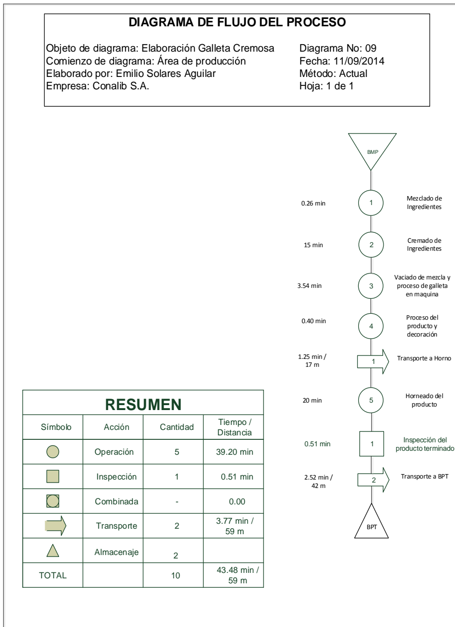
Figura 13. Diagrama de flujo actual de la elaboración de galleta cremosa
