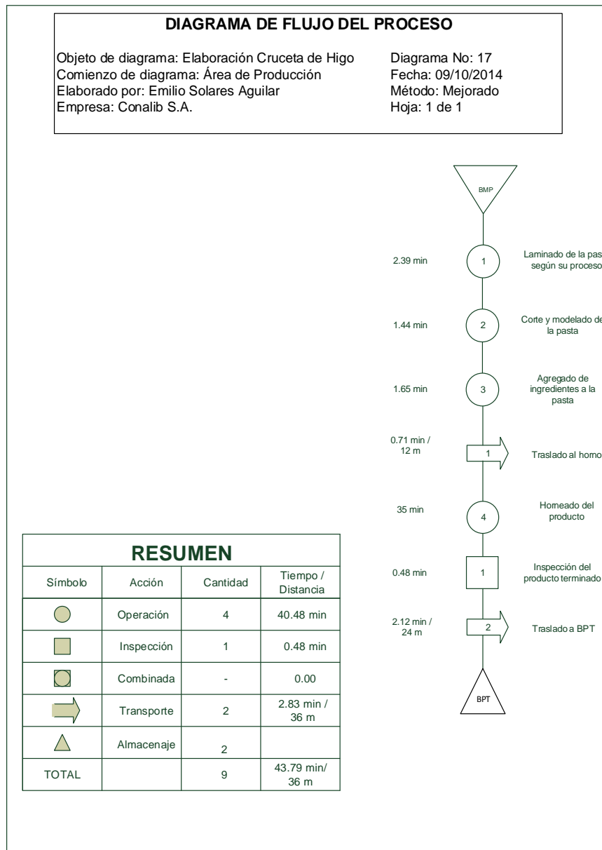
Figura 85. Diagrama de flujo mejorado para la elaboración cruceta de higo
