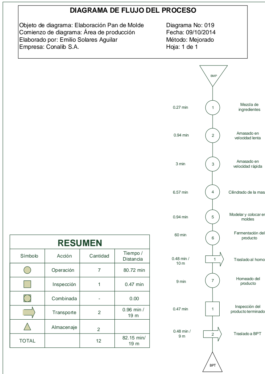
Figura 95. Diagrama de flujo mejorado para la elaboración de pan de molde
