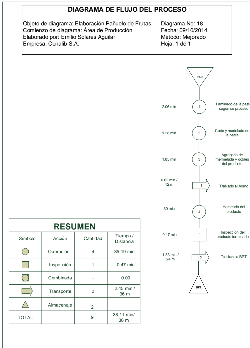
Figura 86. Diagrama de flujo mejorado para la elaboración pañuelo de frutas
