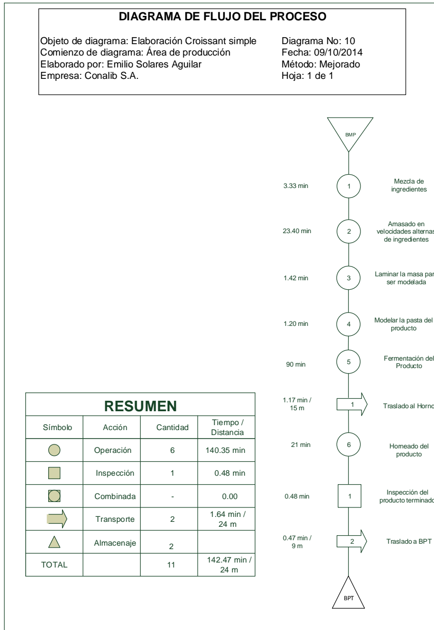
Figura 66. Diagrama de flujo mejorado para la elaboración de croissant simple
