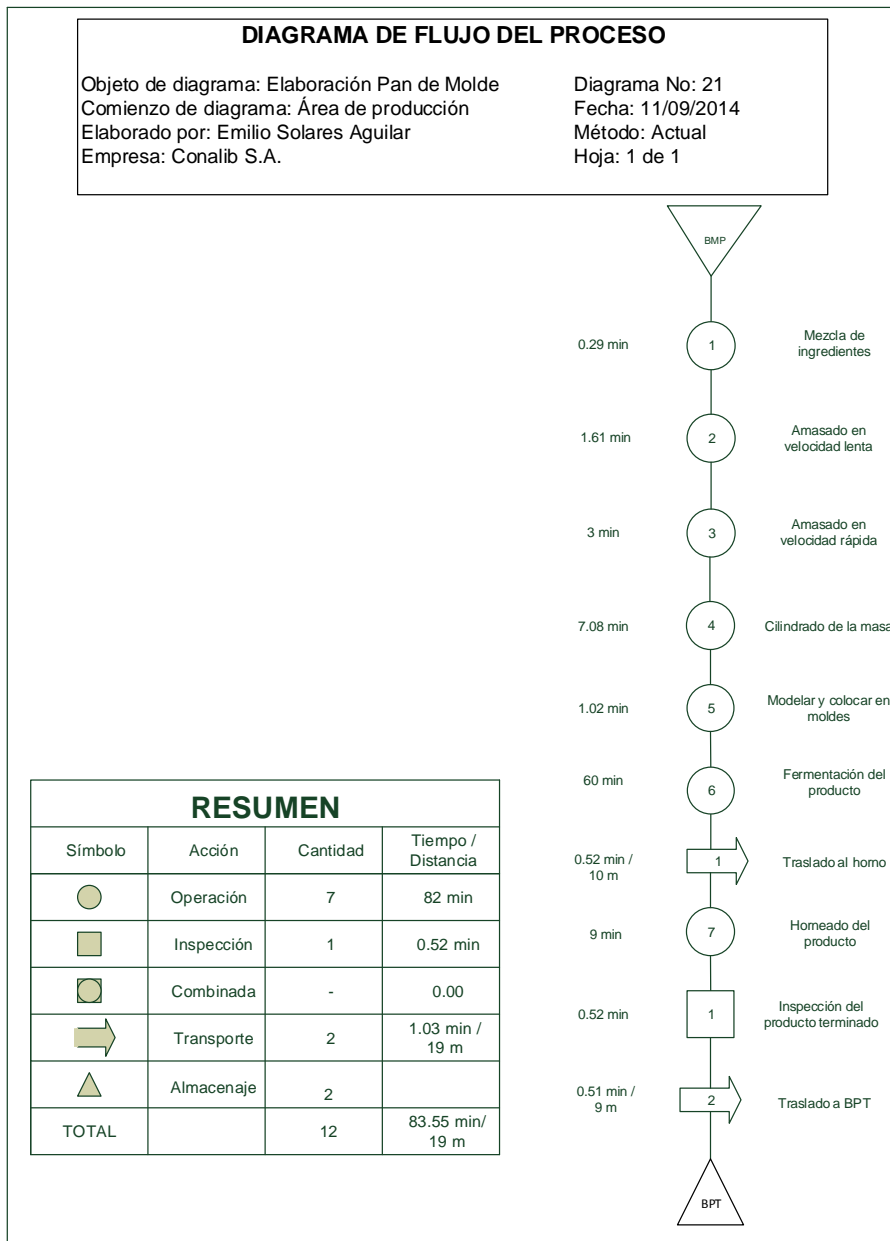
Figura 29. Diagrama de flujo actual de la elaboración de pan de molde
