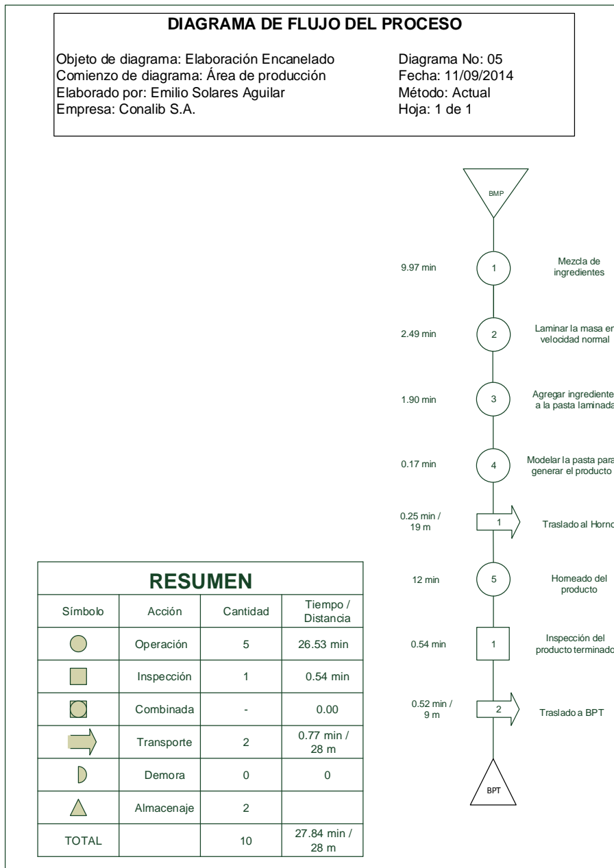
Figura 8. Diagrama de flujo actual de la elaboración de encanelado
