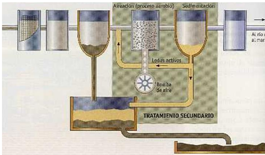
Figura 40. Líneas de tratamiento en las EDAR
