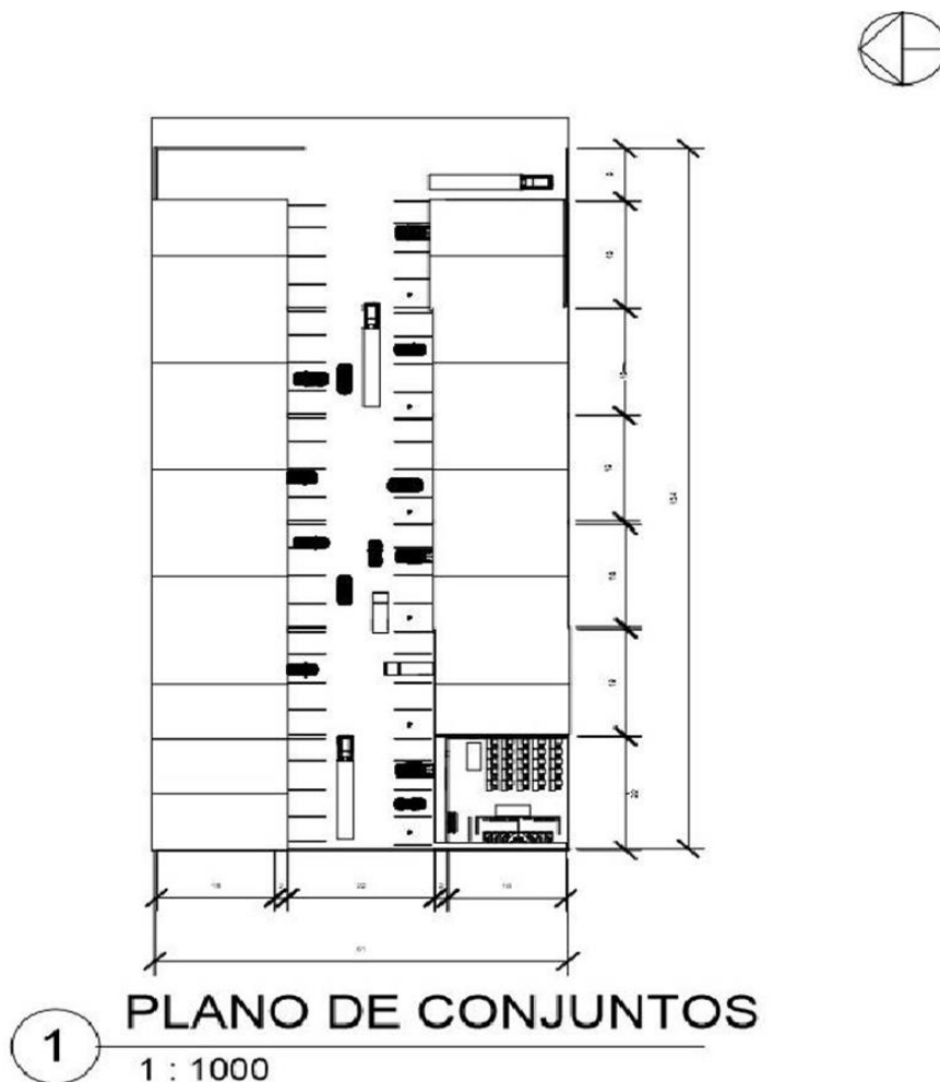
Figura 26. Planos de plantas de producción proyectados hacia el parque industrial en el municipio de San Pedro Sacatepéquez
