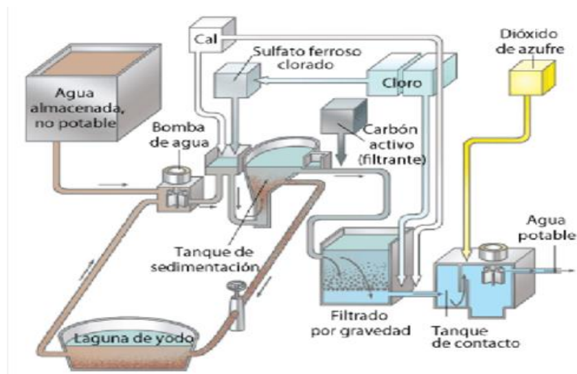
Figura 39. Potabilizadoras de agua, últimas tecnologías para aguas puras
