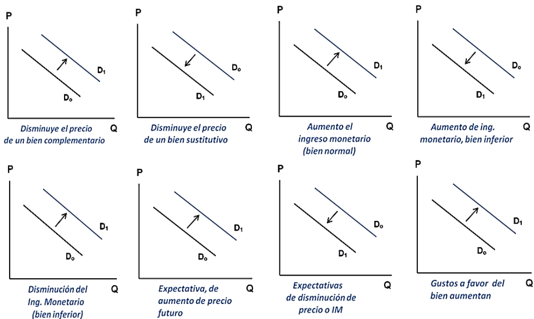
Figura 22. Método geométrico del cambio en la oferta
