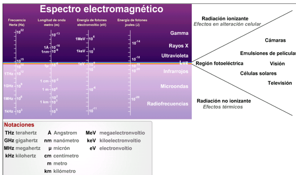
Figura 38. Espectro electromagnético
