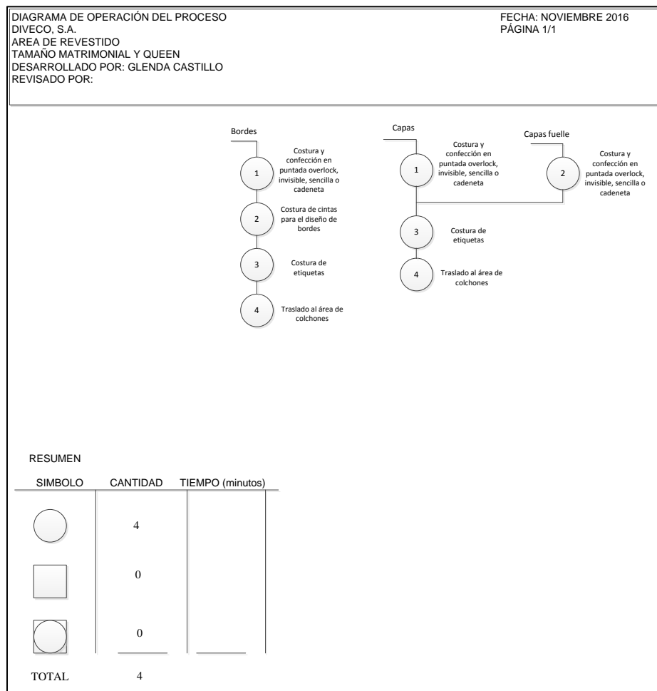
Figura 4. Diagrama de operación del área de revestido
