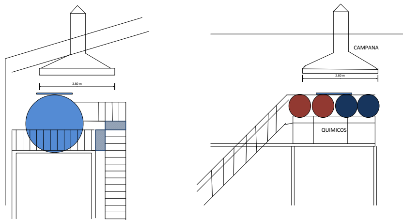
Figura 23. Diseño propuesto del sistema de extracción de gases del área de compactado de esponja
