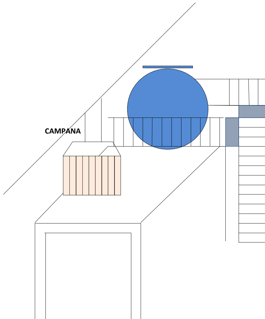
Figura 16. Sistema de extracción de gases actual de compactado de esponja
