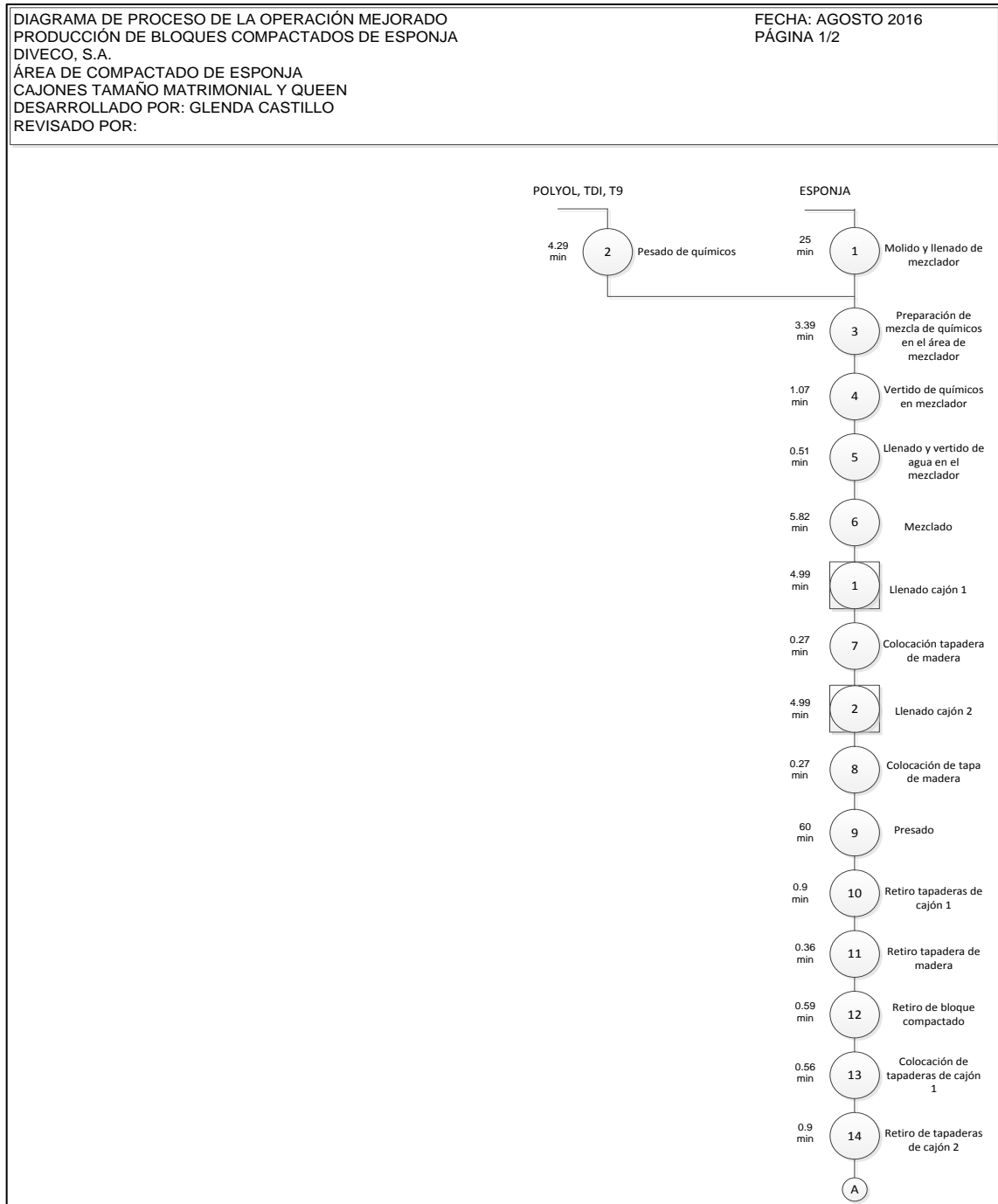
Figura 33. Diagrama mejorado de operaciones del proceso de compactado de esponja para el tamaño Queen y Matrimonial
