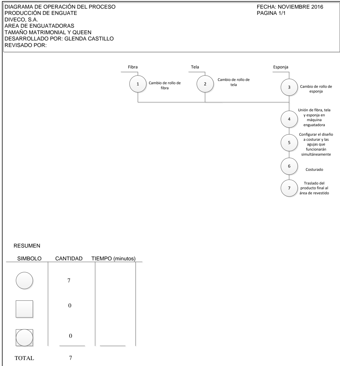
Figura 3. Diagrama de operación del proceso de enguate
