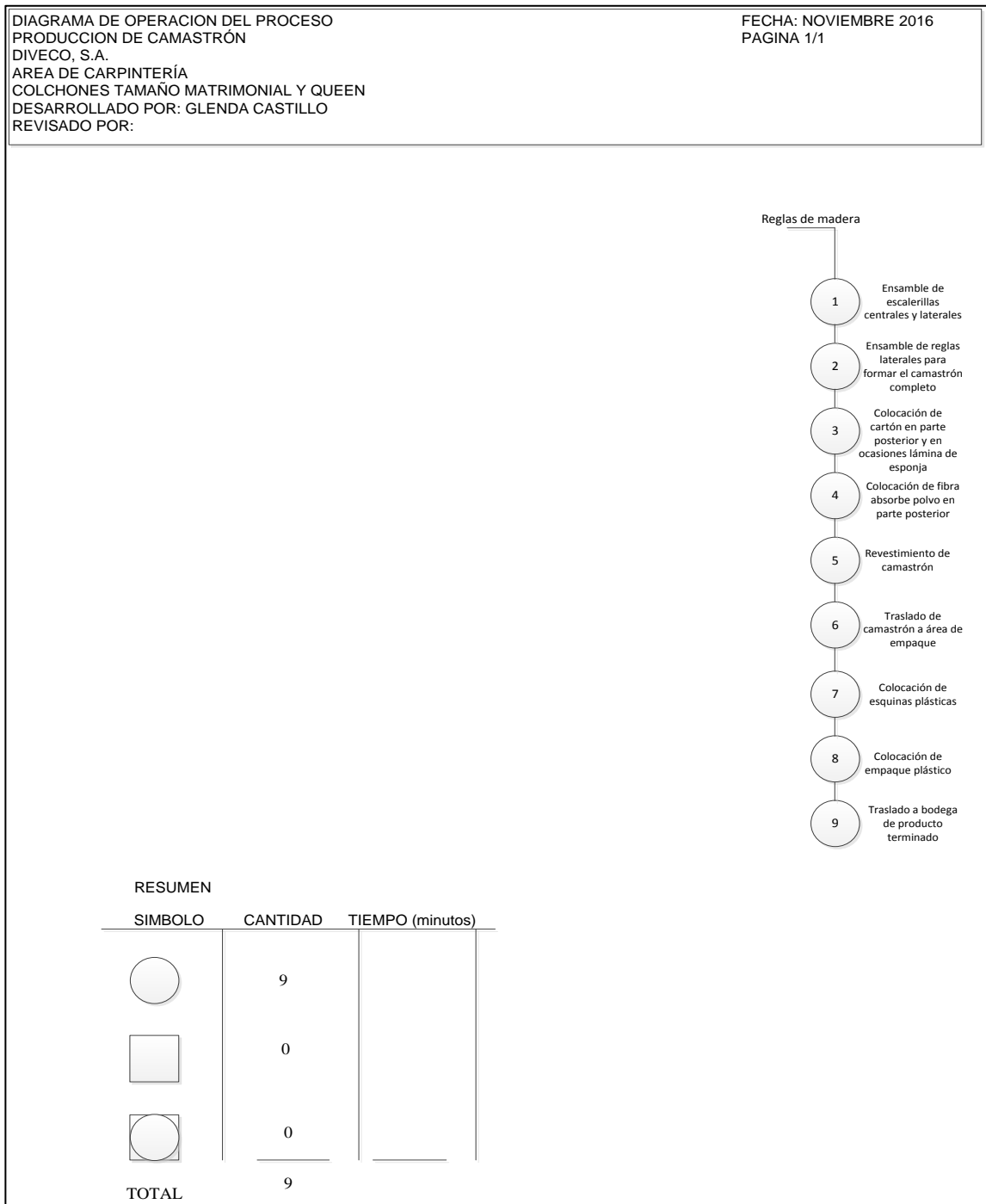
Figura 6. Diagrama de operaciones del área de carpintería
