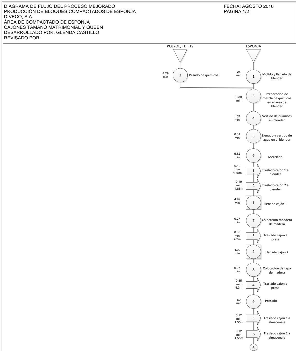
Figura 35. Diagrama mejorado de flujo del proceso de compactado de esponja para el tamaño queen y matrimonial
