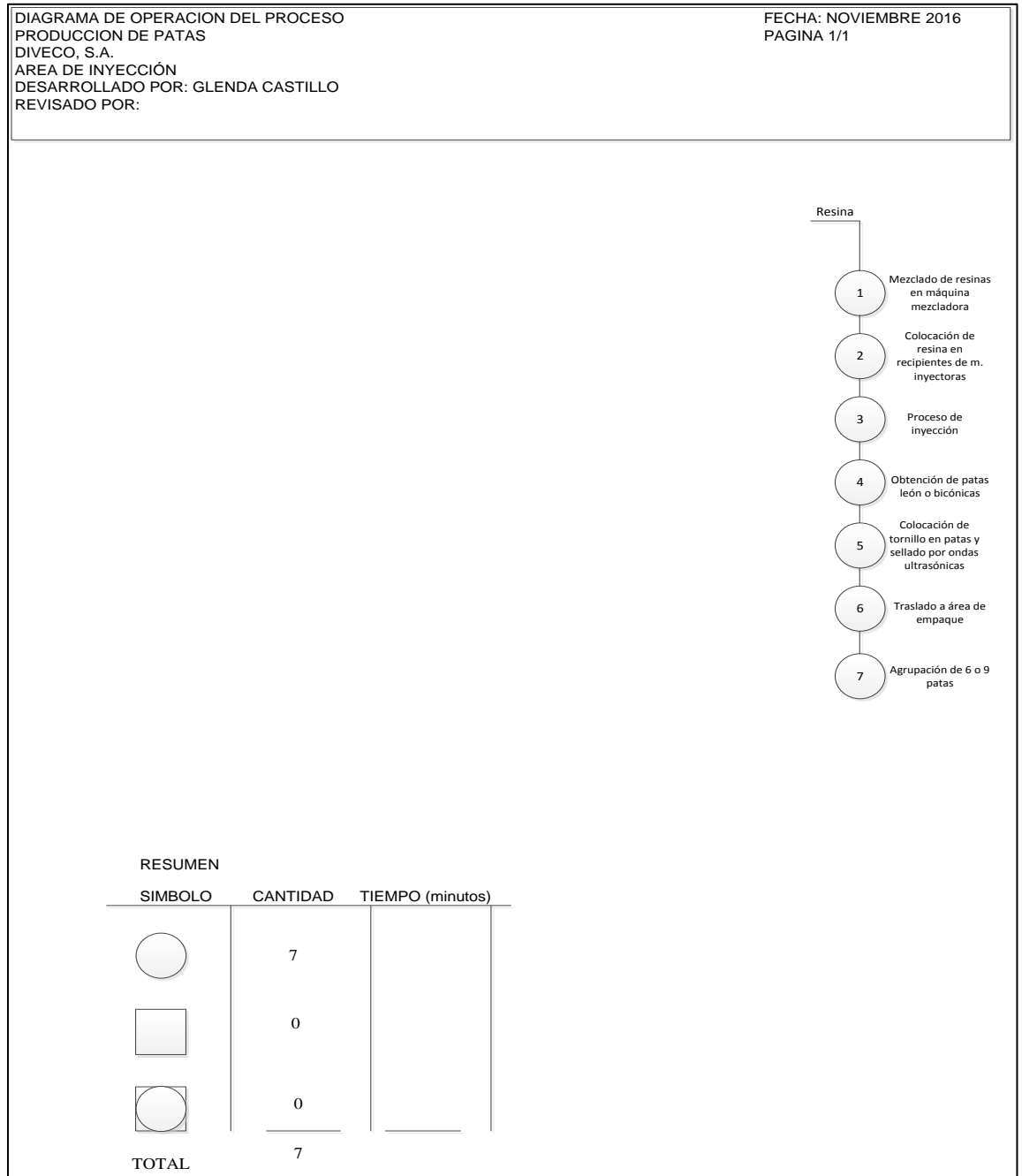
Figura 8. Diagrama de operación del área de inyección
