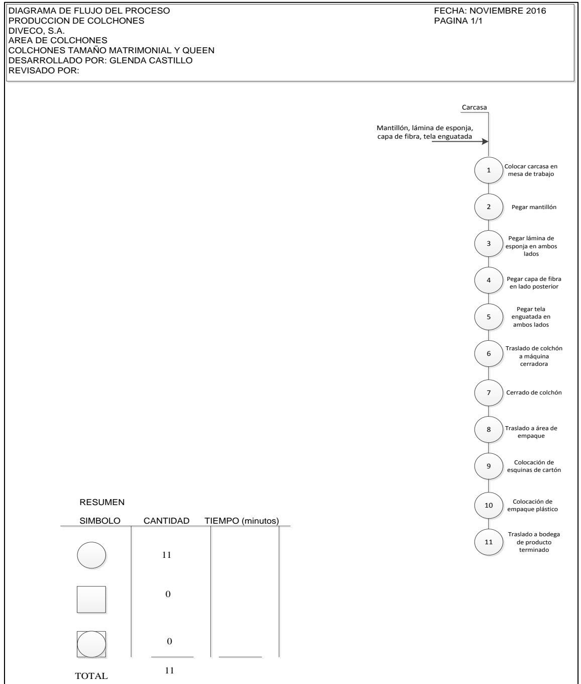
Figura 5. Diagrama de operación del área de colchones
