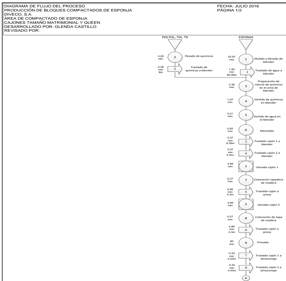
Figura 29. Diagrama de flujo del proceso estandarizado del área de compactado de esponja para el tamaño queen y matrimonial
