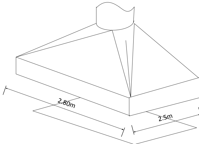
Figura 22. Diseño con dimensiones del sistema de extracción
