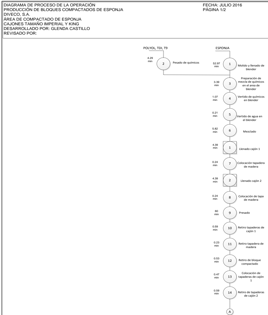
Figura 28. Diagrama de proceso de la operación estandarizado del área de compactado de esponja para el tamaño imperial y king
