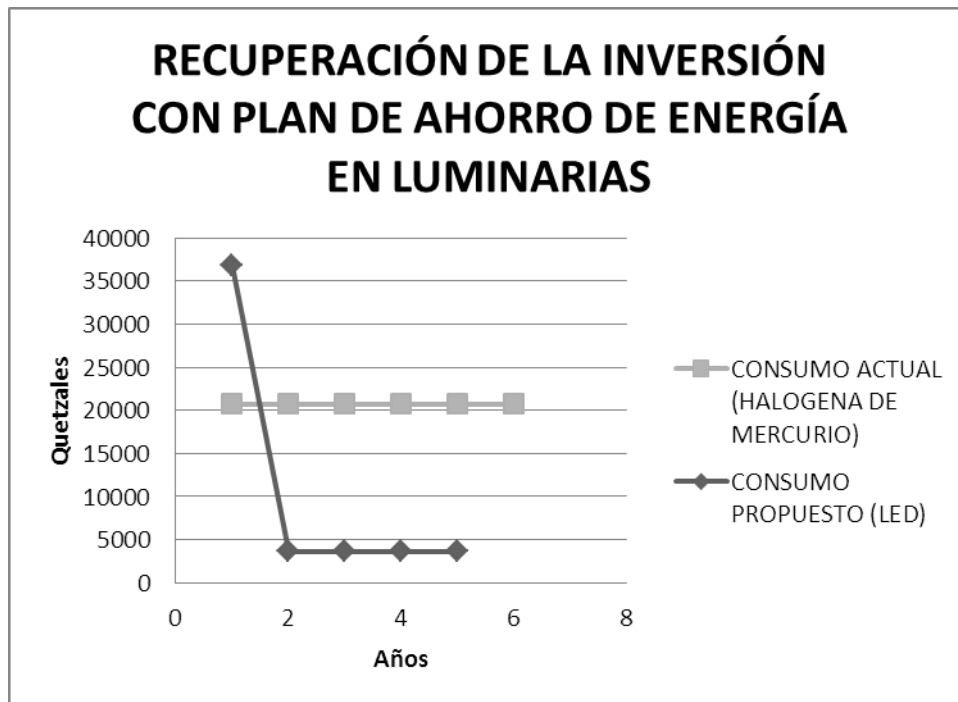
Figura 40. Gráfica de tiempo estimado de recuperación de la inversión económica de la propuesta de ahorro de energía
