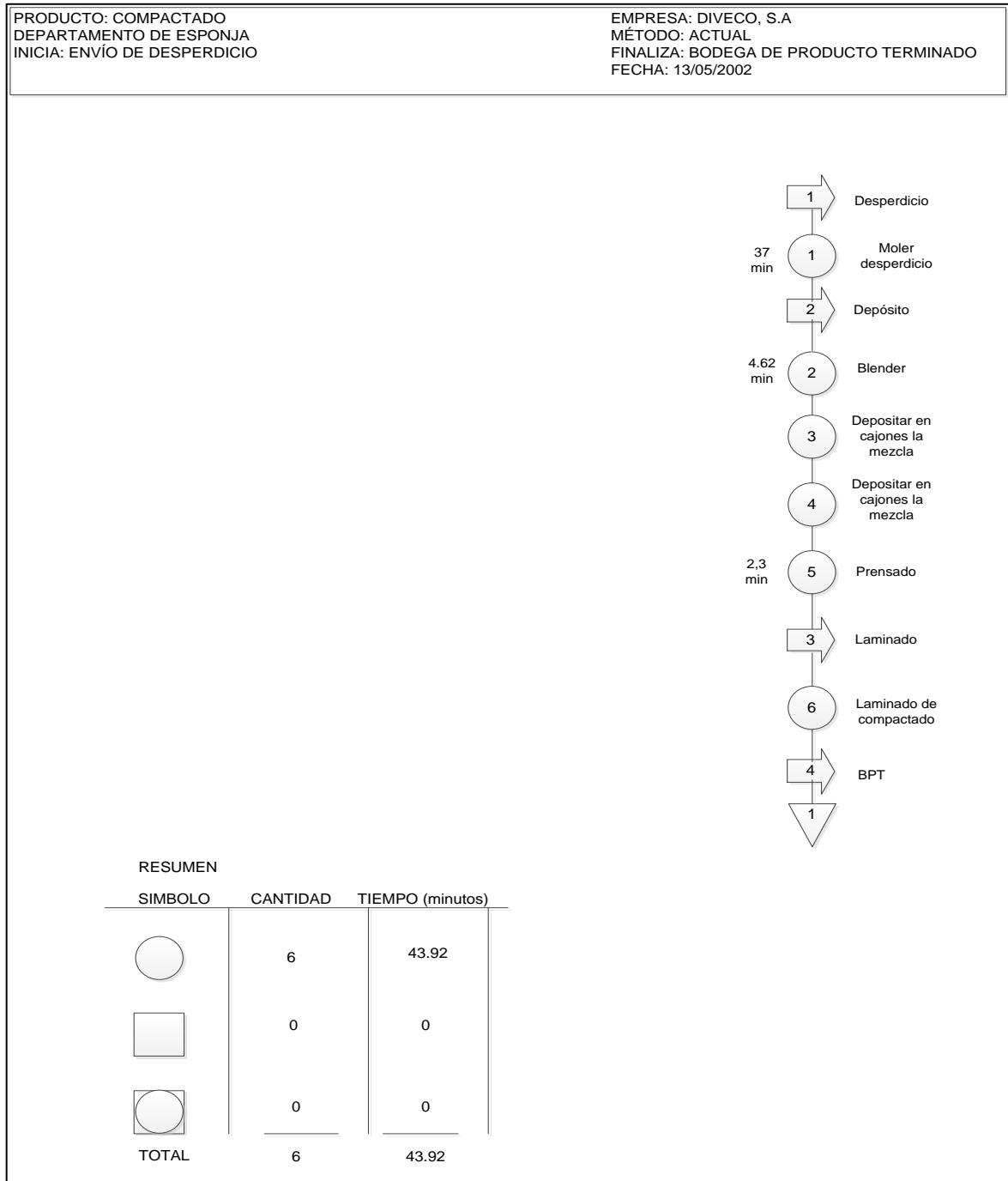
Figura 18. Diagrama de flujo del proceso del área de compactado de esponja
