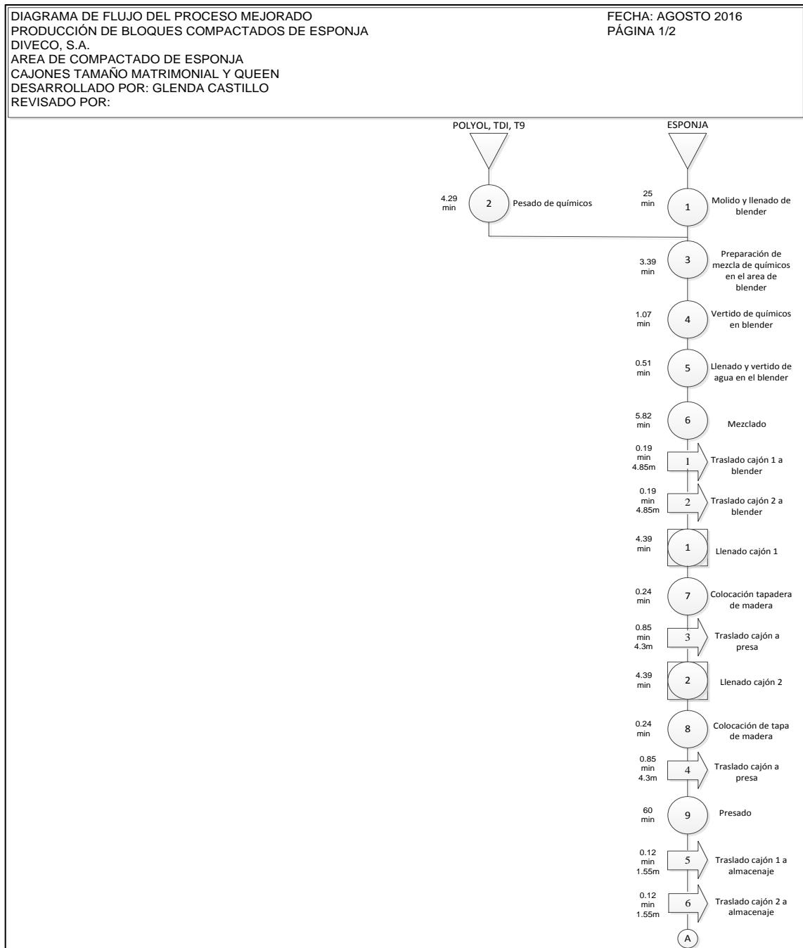
Figura 36. Diagrama mejorado de flujo del proceso de compactado de esponja para el tamaño imperial y king
