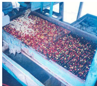
Figura 15. Zarandas oscilantes
