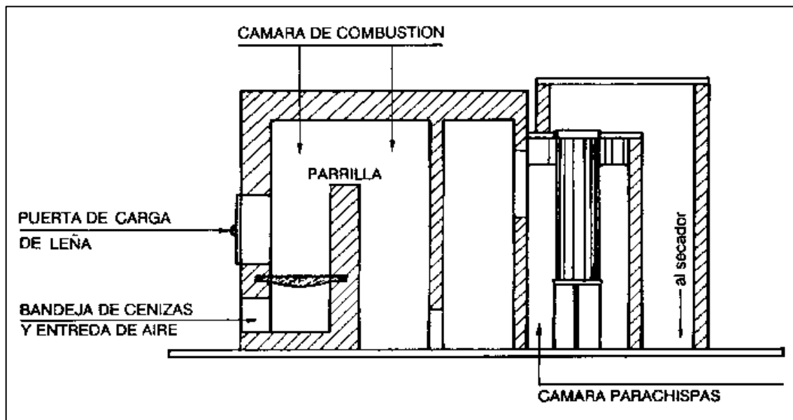
Figura 29. Horno de fuego directo
