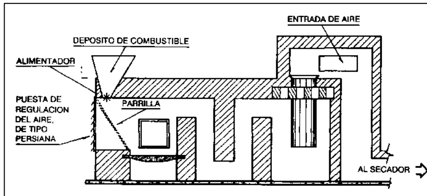
Figura 23. Horno calorífico
