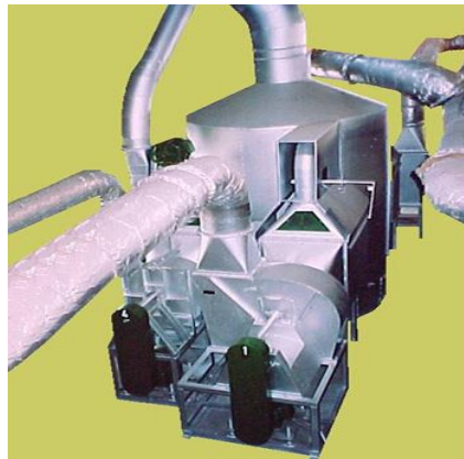
Figura 27. Horno múltiple
