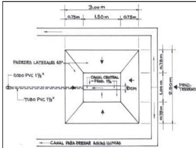
Figura 59. Vista superior del cobertizo
