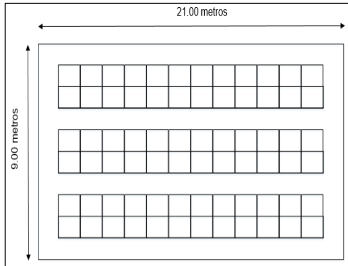
Figura 62. Dimensiones de secador solar
