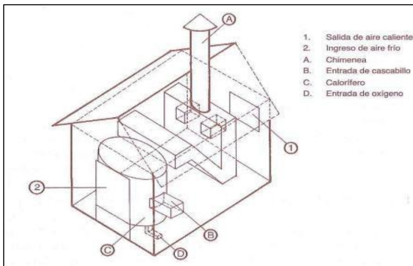
Figura 28. Horno mejorado con inyección de oxígeno
