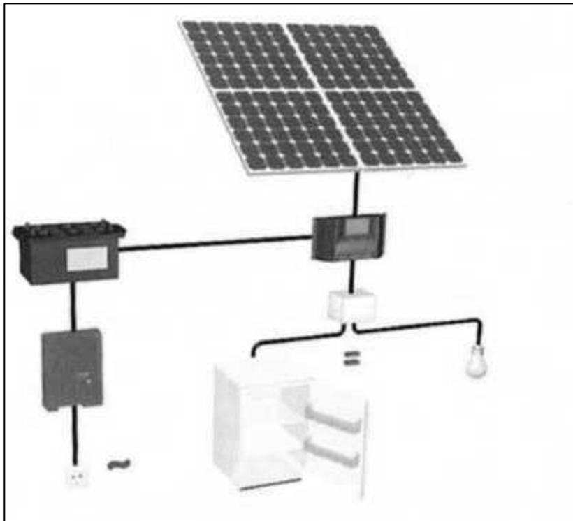
Figura 68. Instalación fotovoltaica aislada de la red
