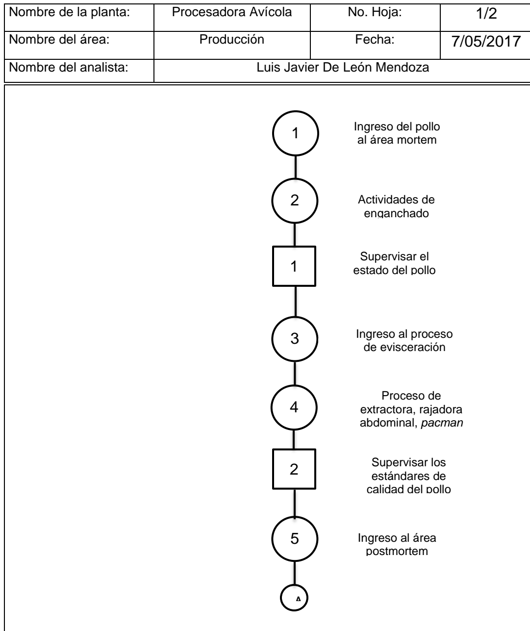
Figura 2. Diagrama de operaciones del proceso correspondiente en la avícola
