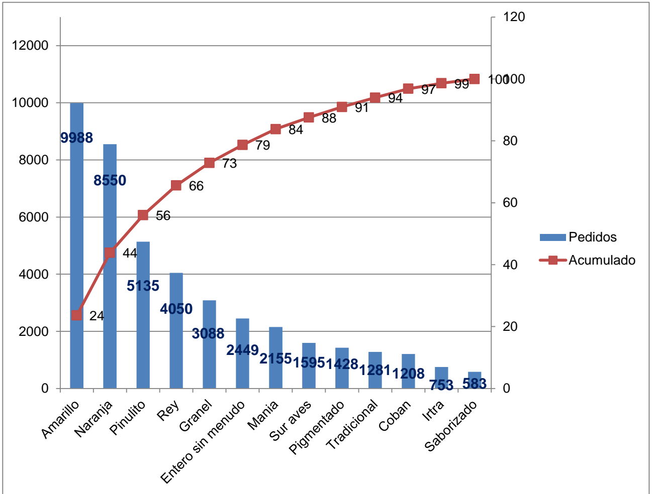
Figura 3. Diagrama de Pareto de las diferentes presentaciones de pollo
