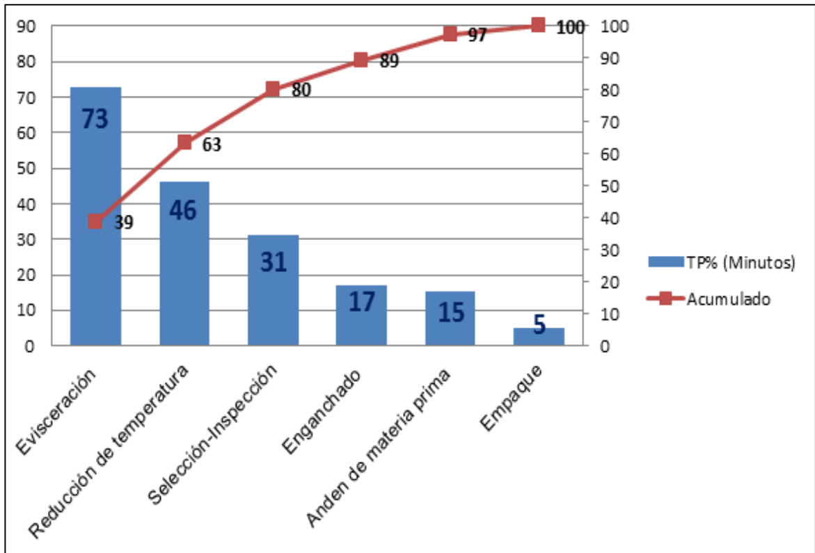
Figura 8. Diagrama de tiempo perdido por paros (semanal)
