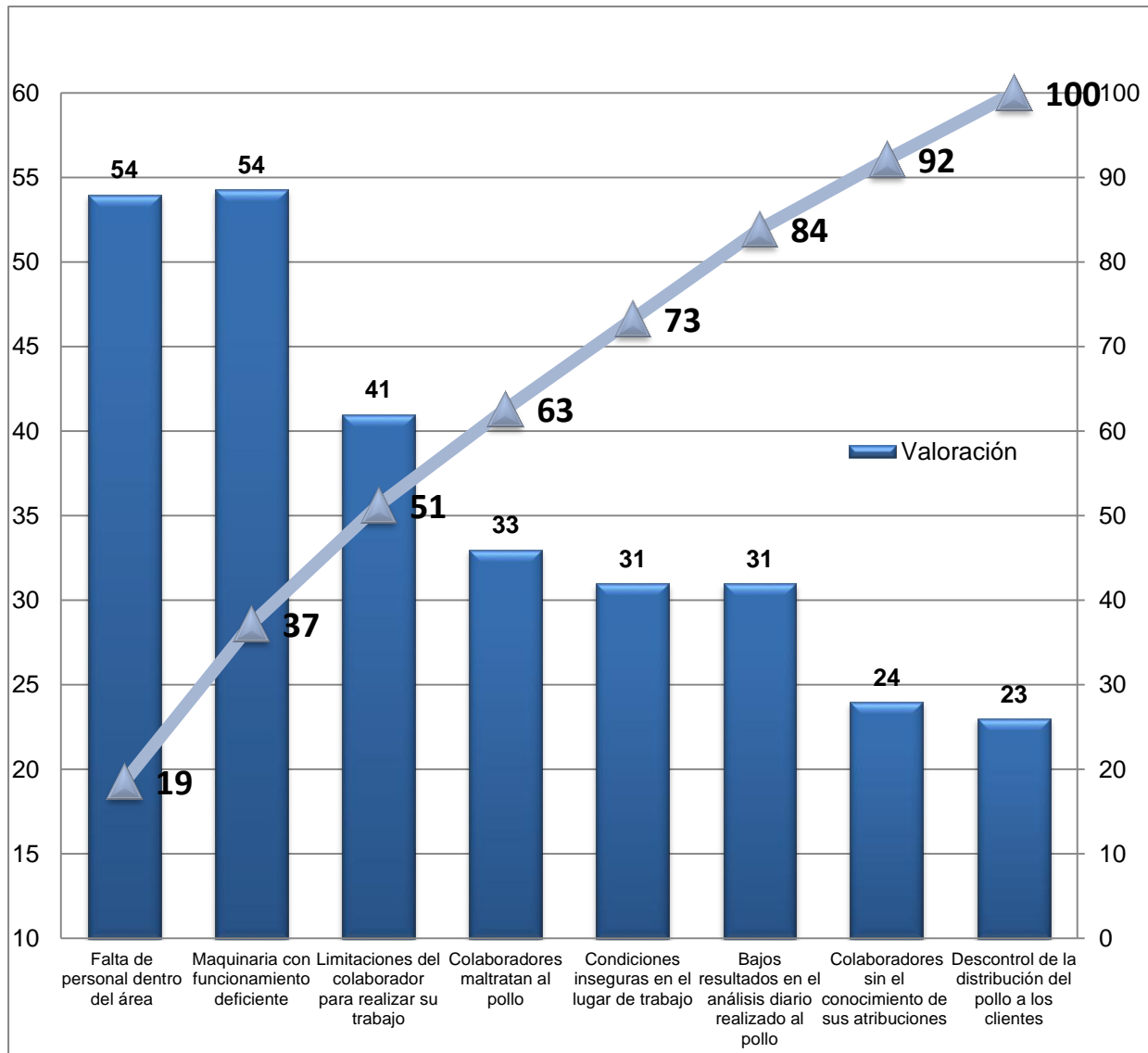
Figura 7. Diagrama de Pareto de los principales problemas en área postmortem
