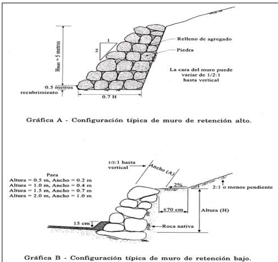
Figura 4. Esquema típico de muros de roca
