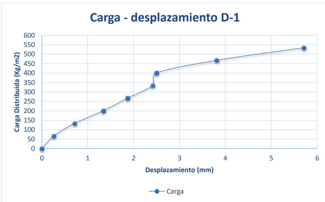
Figura 44. Gráfica del comportamiento carga-deformación en la unión de la viga de bambú que une el sistema bambú-ferrocemento, aplicándole el 100 por ciento de carga adicional a la carga de diseño
