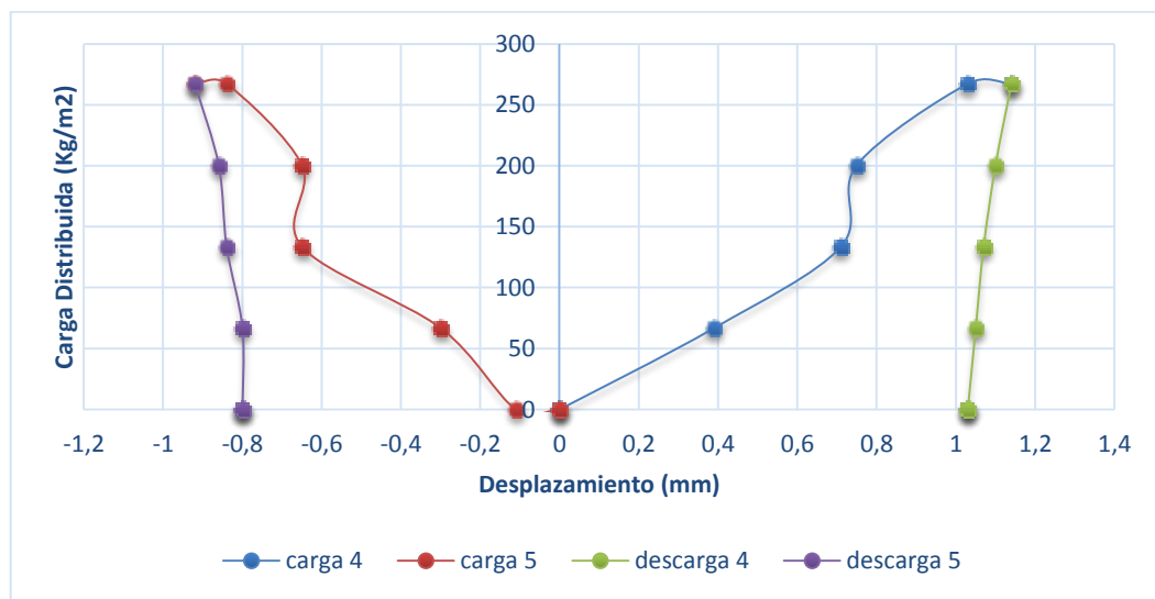
Figura 42. Carga - desplazamiento D-4 y D-5
