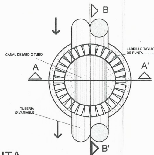
PLANTA ESCALA 1/50
