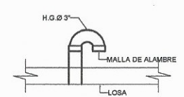
DETALLE DE TUBO DE VENTILACION
