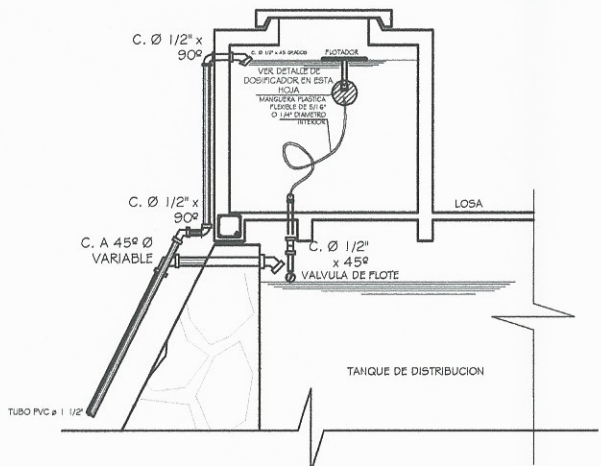
SECCION A-A' DE HIPOCLORADOR
