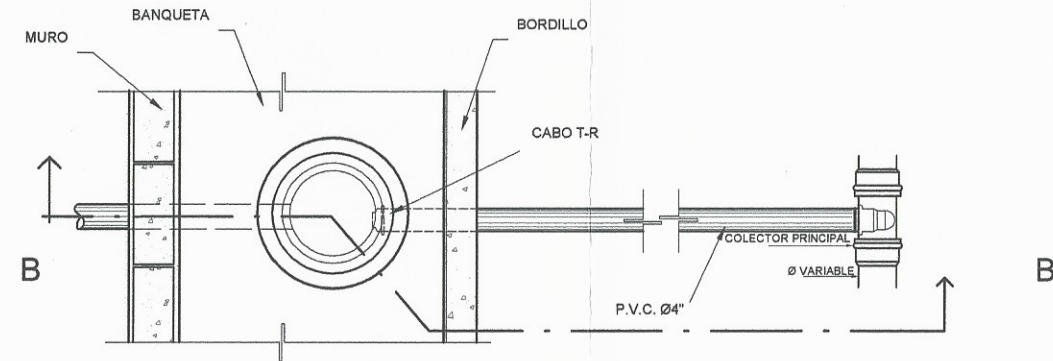
PLANTA ESCALA 1/15
