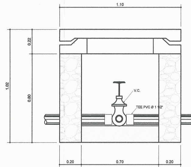
SECCIÓN B-B' VÁLVULA DE LIMPIEZA
