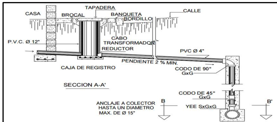
Figura 3. Conexiones domiciliarias
