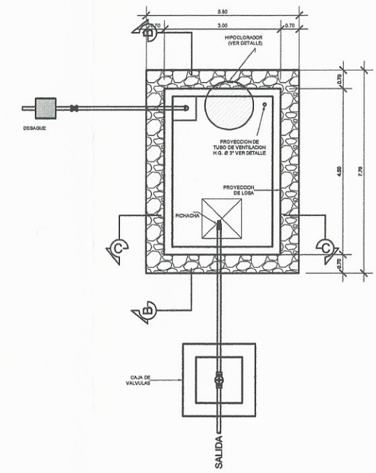
PLANTA DE TANQUE DE DISTRIBUCION
