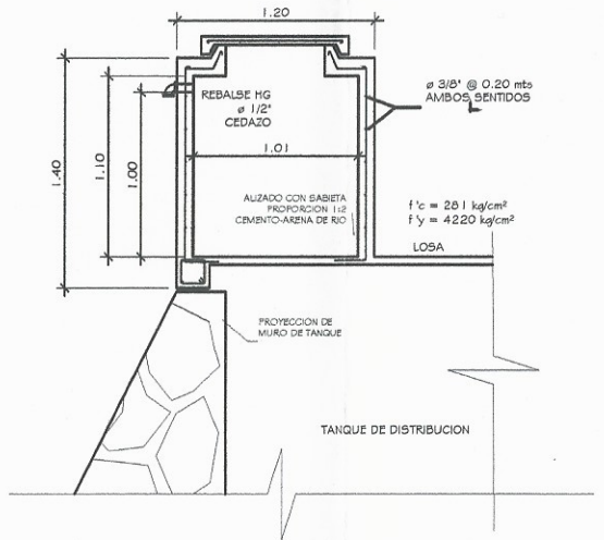
DETALLE DE ARMADO
