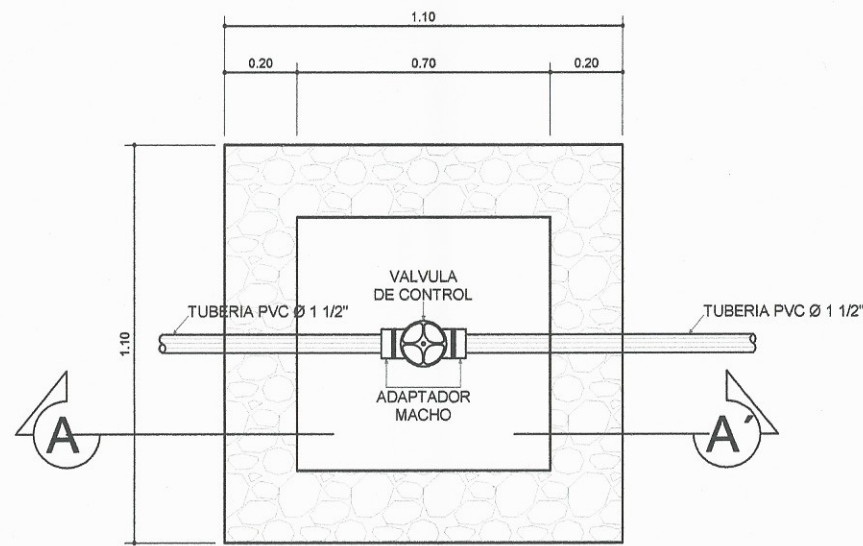
PLANTA VÁLVULA DE COMPUERTA
