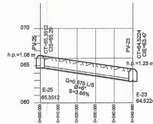
PERFIL PV-25 A PV-23
