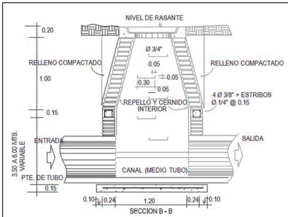
Figura 2. Partes de un pozo de visita
