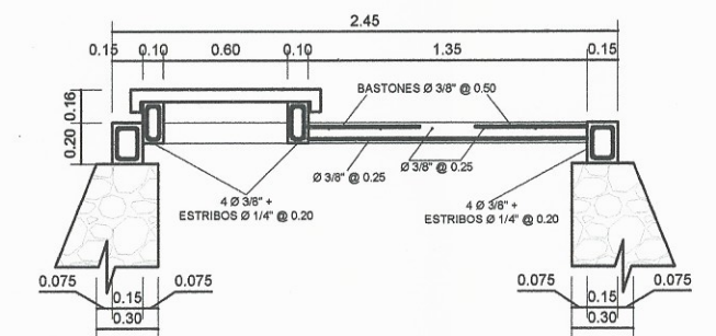
SECCION E-E' DE TANQUE
