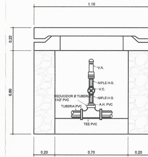
SECCIÓN C-C' VÁLVULA DE AIRE
