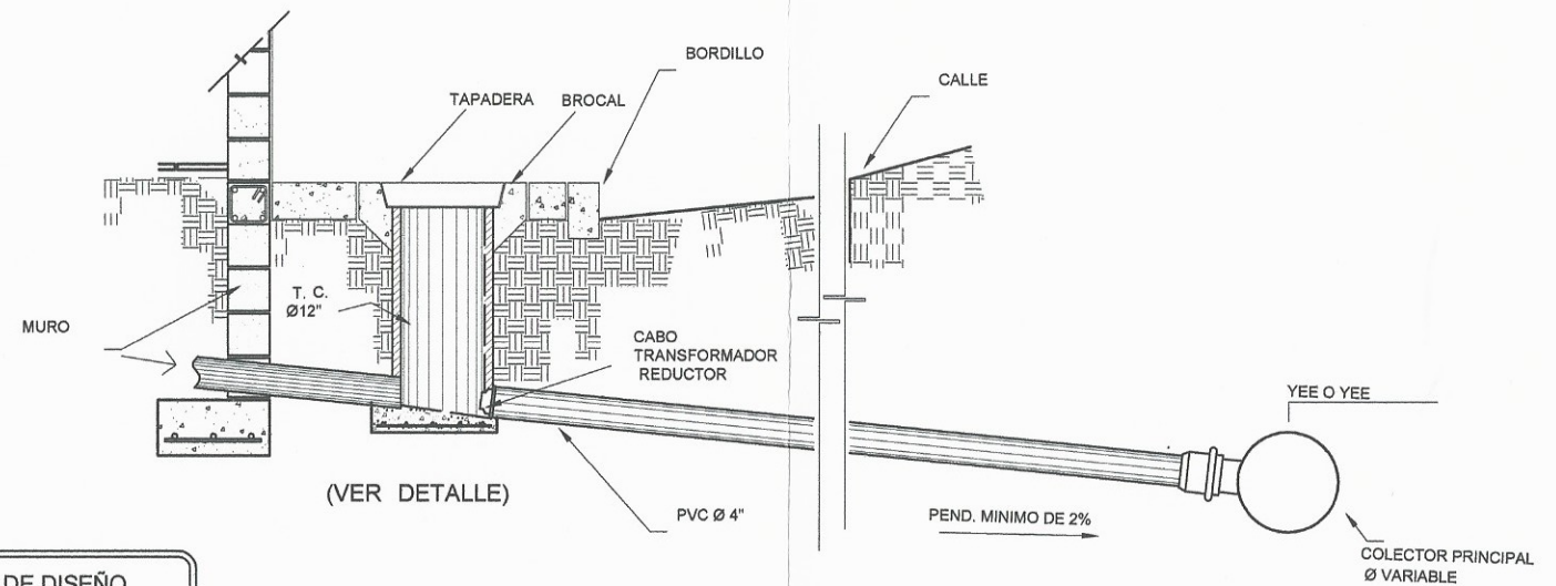
SECCION B-B' ESCALA 1/15
