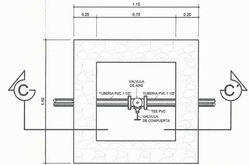
PLANTA VÁLVULA DE AIRE
