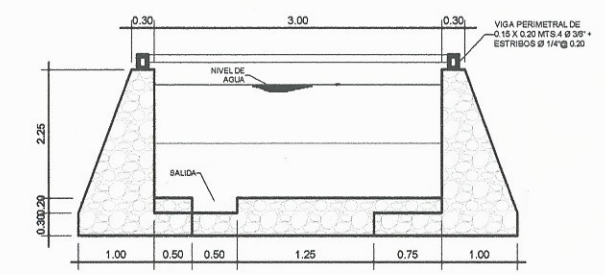
SECCION C-C DE TANQUE
