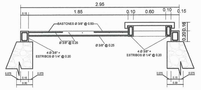
SECCION D-D' DE TANQUE
