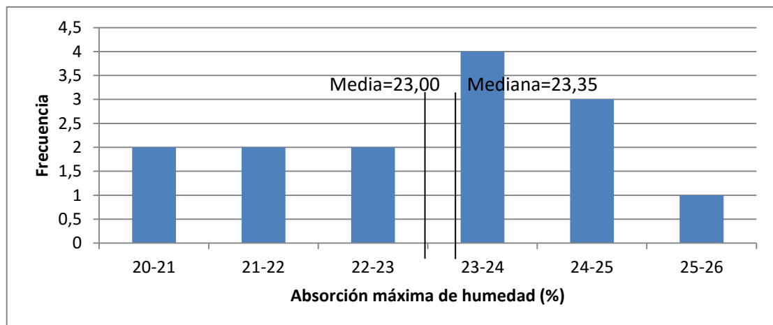
Figura 10. Histograma de frecuencias agrupadas: absorción de humedad (corregido)
