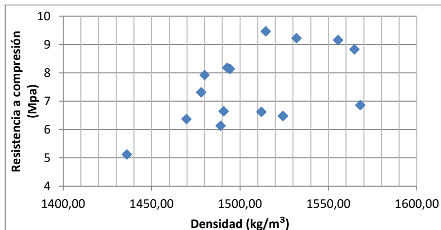
Figura 6. Resistencia a compresión como función de la densidad
