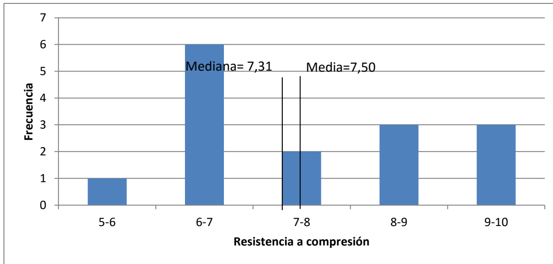
Figura 8. Histograma de frecuencias agrupadas: resistencia a compresión (corrección)
