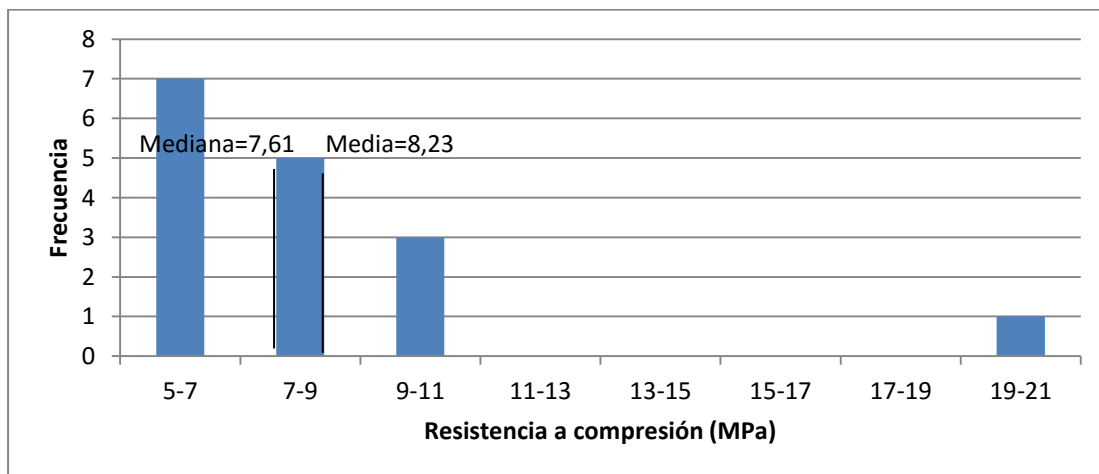
Figura 7. Histograma de frecuencias agrupadas: resistencia a compresión
