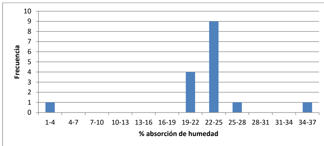
Figura 9. Histograma de frecuencias agrupadas: absorción de humedad
