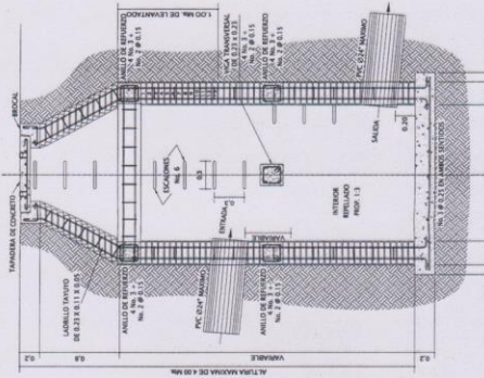
SECCION POZO (1.25 MTS) H = 0-4 MTS. ESC. 1/50
