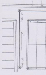
PLANTA PV-DS-23 A PV-DS-24 ESC. 1:50 TAMAÑO 5
