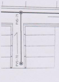
PLANTA PV-DS-70 A PV-DS-71 TRAMO 24 ESC. 1/500
