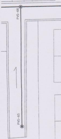
PLANTA PV-DS-65 A PV-DS-66 TRAMO 22 ESC. 1/500
