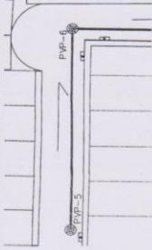
PLANTA PV-DP-5 A PV-DP-6 TRAMO 2 E.C. 1: 500
