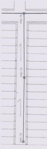
PLANTA PV-DS-72 A PV-DS-74 TRAMO 25 ESC. 1/500
