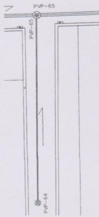
PLANTA PV-DP-64 A PV-DP-65 TRAMO 21 ESC. 1000
