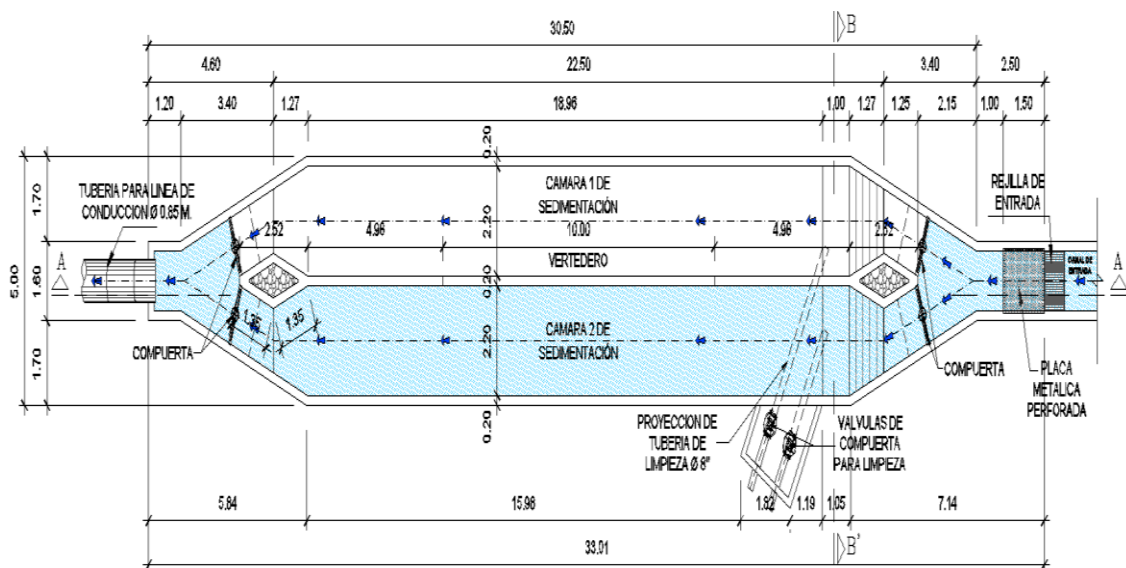
Figura 11. Planta desarenador hidroeléctrica Cholivá
