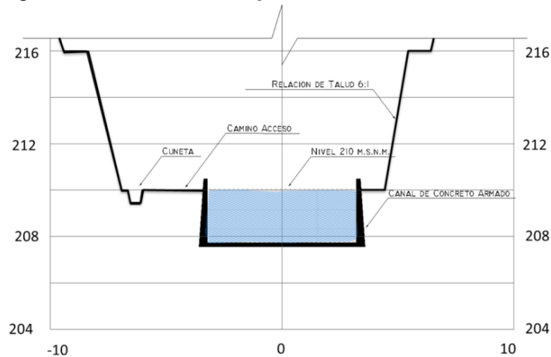
Figura 12. Sección típica de canal de conducción
