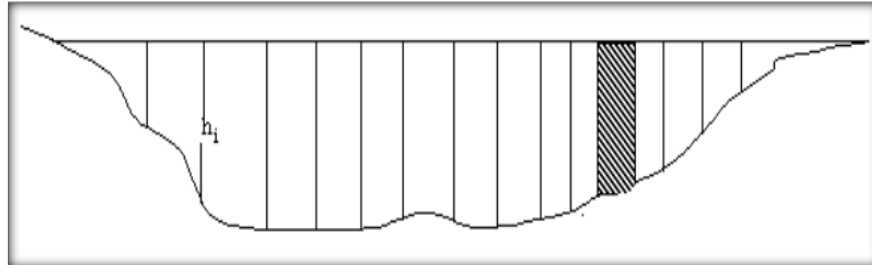
Figura 19. Sección transversal para el método área velocidad
