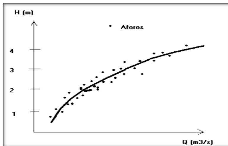
Figura 18. Gráfica de descarga altura contra caudal
