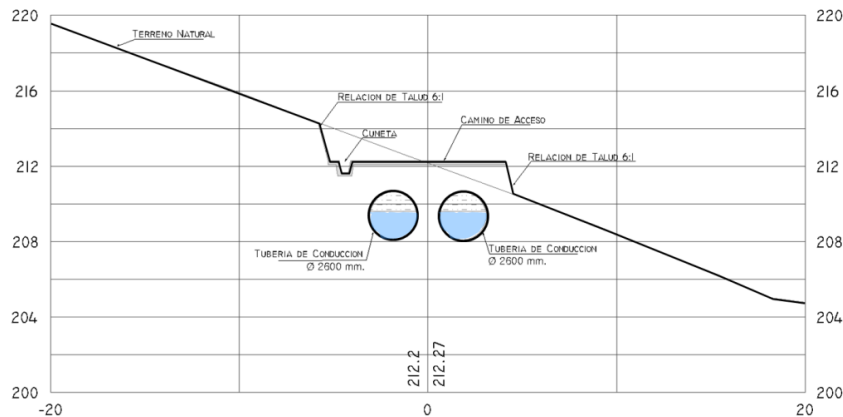
Figura 13. Tubería de conducción
