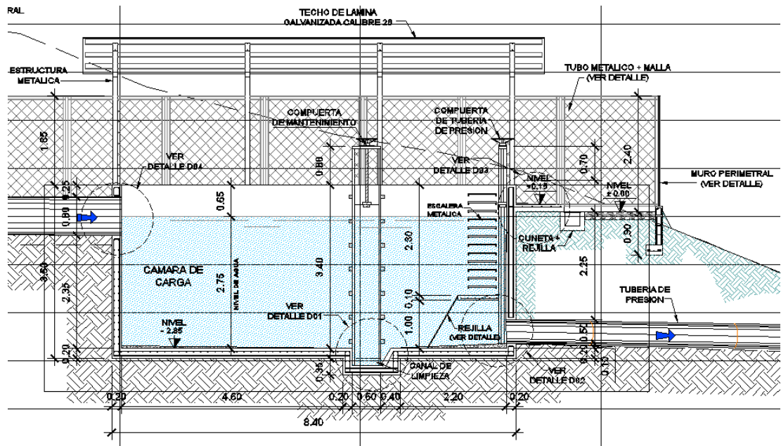
Figura 14. Perfil de cámara de carga hidroeléctrica Cholivá
