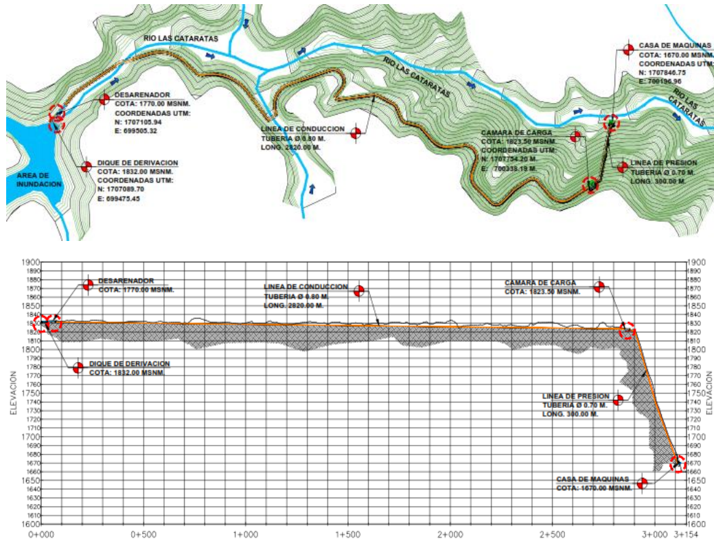
Figura 17. Planta y perfil general de una central hidroeléctrica
