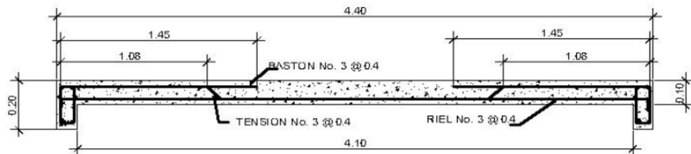
DETALLE No. 1 ARMADO DE LOSA ESCALA V. 1/10 ESCALA H. 1/20
