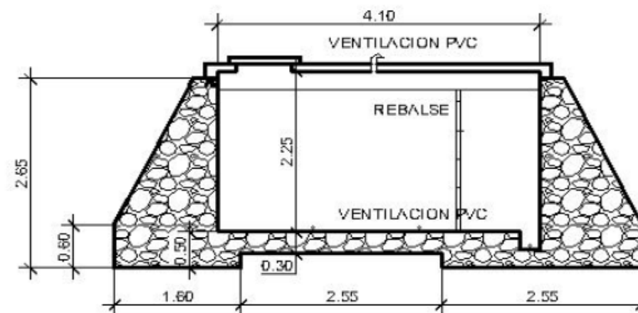
SECCION B-B' TANQUE DE DISTRIBUCION ESCALA 1/50
