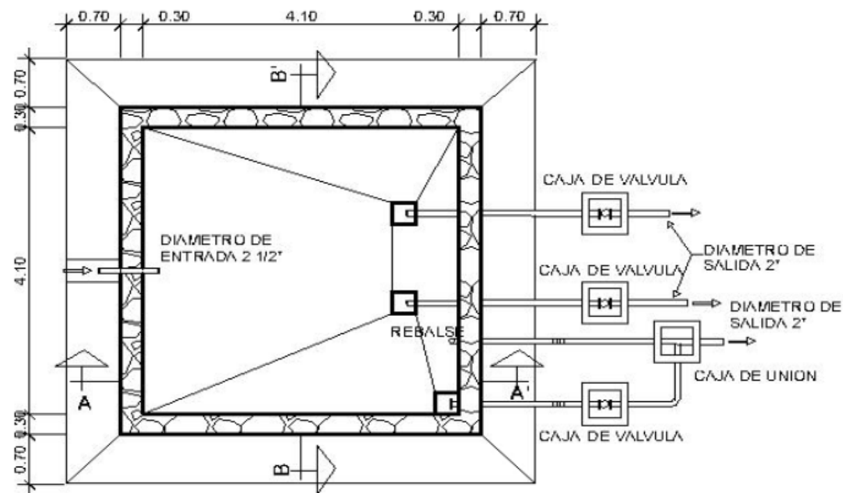
PLANTA TANQUE DE DISTRIBUCION ESCALA 1/50
