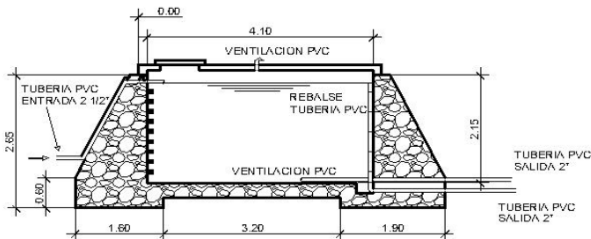
SECCION A-A' TANQUE DE DISTRIBUCION ESCALA 1/50
