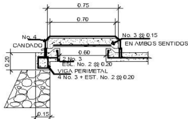
DETALLE No. 1 TAPADERA ESCALA 1/15
