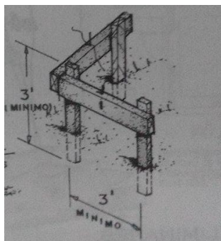
Figura 7. Colocación de puente
