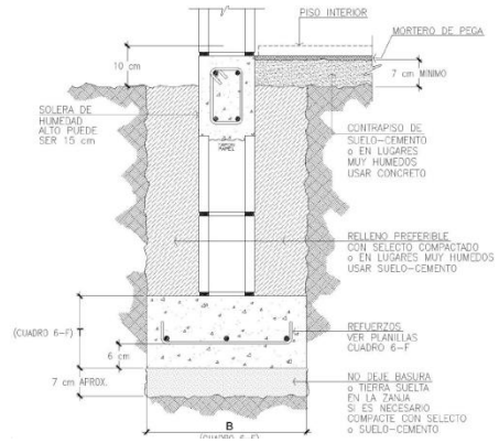
Figura 6. Detalle de la configuración del cimiento corrido
