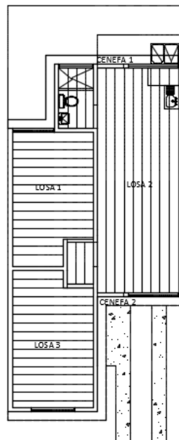
Figura 18. Orientación de entarimado
