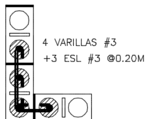
Figura 21. Detalle de refuerzo tipo A
