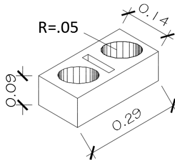
Figura 20. Detalle de ladrillo tubular
