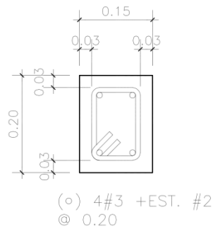
Figura 11. Sección de soleras
