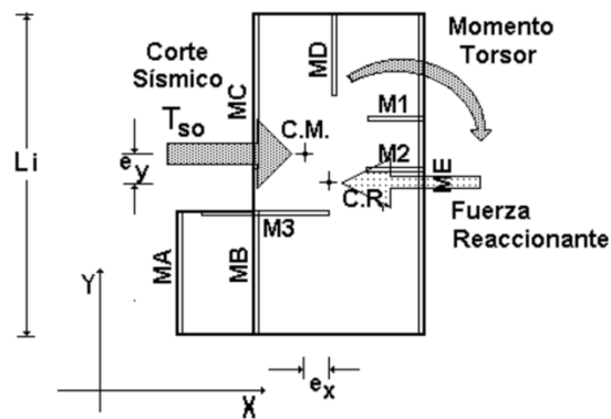
Figura 3. Planta de vivienda con poca rigidez torsional
