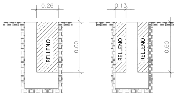
Figura 9. Sección de relleno compactado
