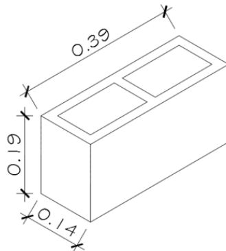
Figura 14. Detalle de block de concreto
