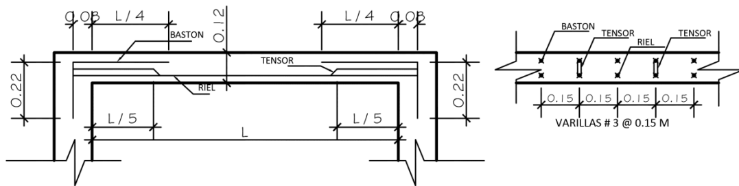
Figura 16. Sección de losas
