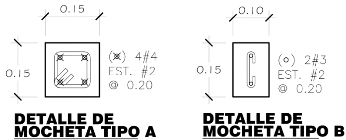
Figura 15. Detalles de mochetas
