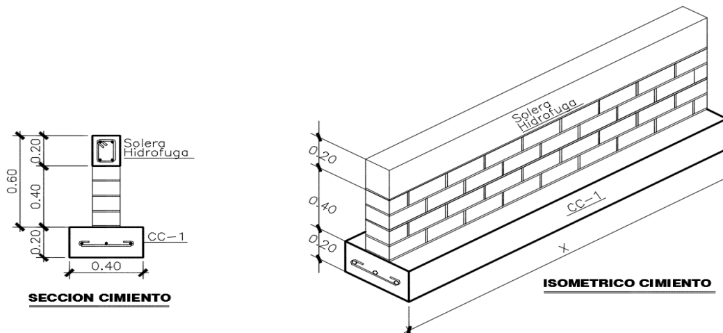
Figura 19. Detalles de cimentación
