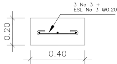
Figura 10. Sección de cimiento corrido
