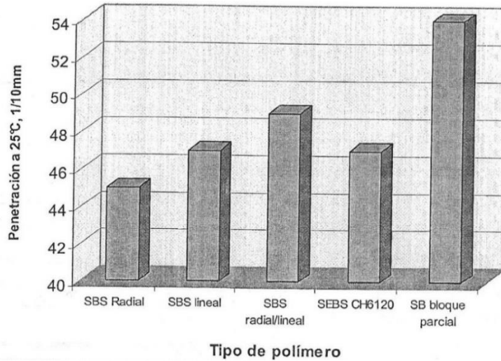
Figura 22. Penetración con diferentes co polímeros de estireno-butadieno.
