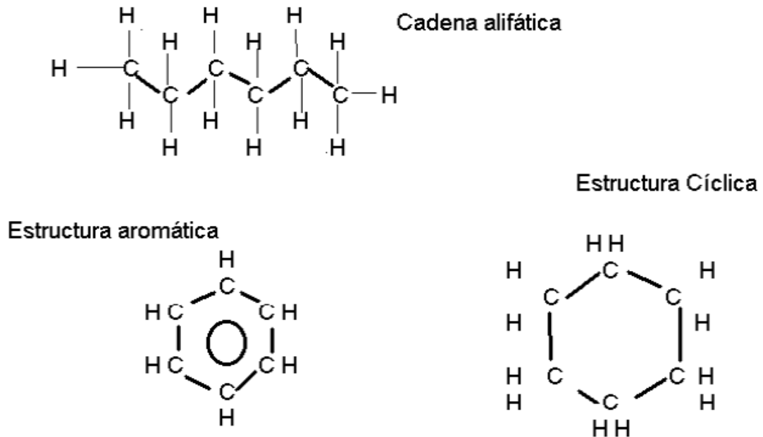
Figura 3. Tipos de moléculas asfálticas
