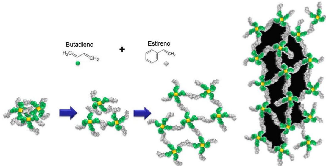
Figura 26. Esquema de modificación de un cemento asfáltico
