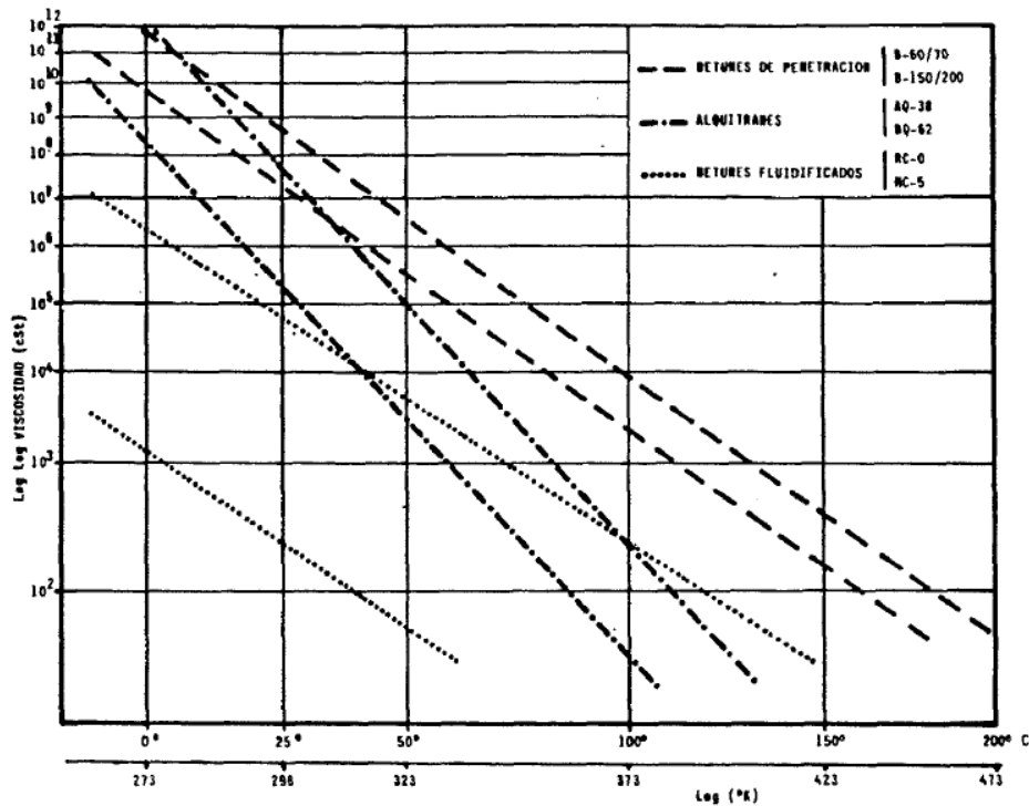
Figura 7. Diagramas de viscosidad- temperatura de diferentes cementos asfálticos
