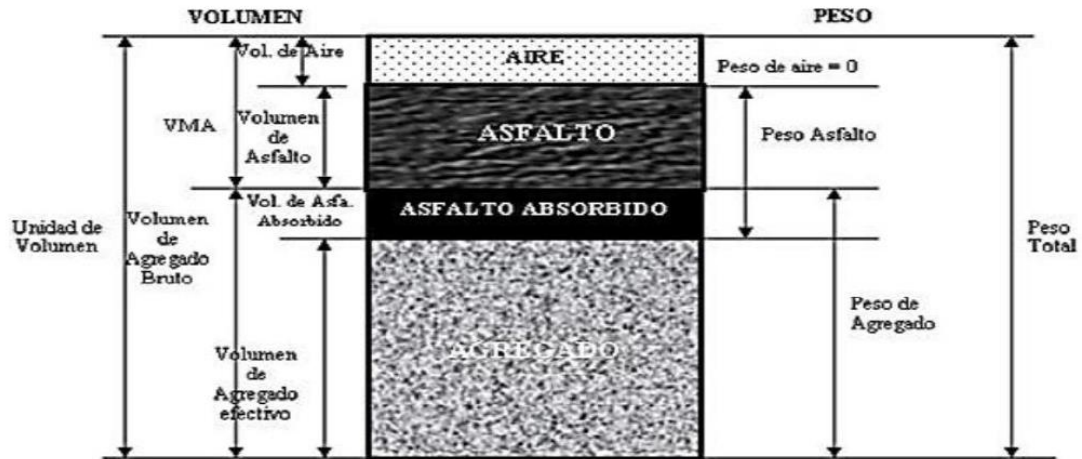
Figura 63. Composición típica de una MAC
