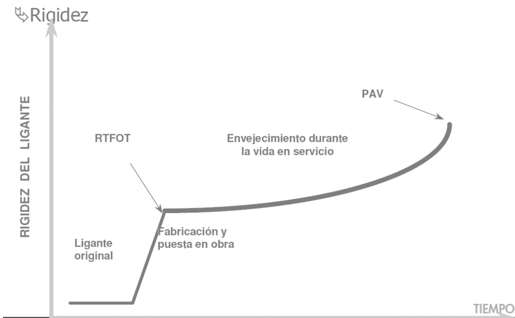
Figura 13. Rigidez de un asfalto
