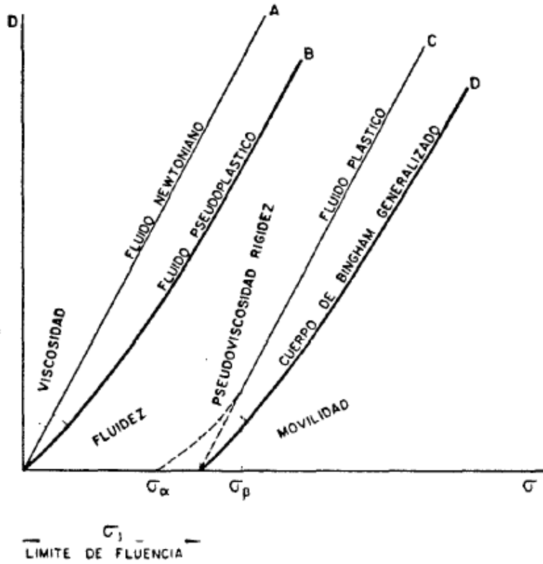
Figura 5. Diagrama reológico
