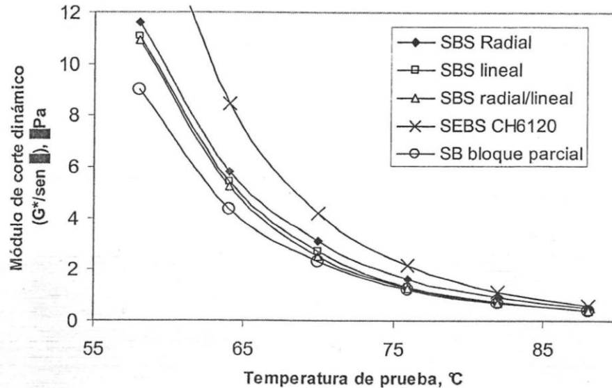
Figura 25. Relación de G'/\text{sen } \delta vs la temperatura de las pruebas
