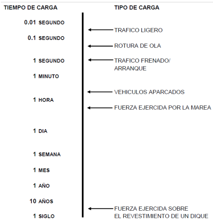
Figura 9. Diferentes tipos de cargas y su tiempo de aplicación
