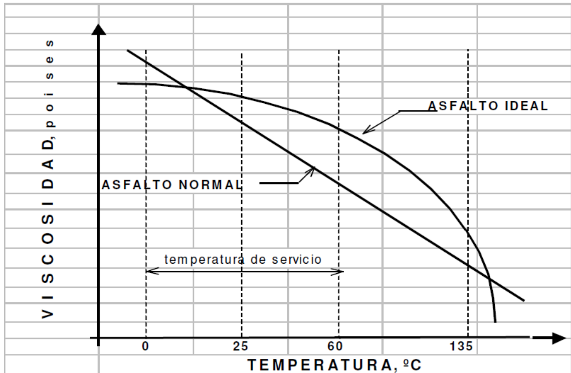
Figura 6. Representación de un “asfalto ideal” desde el punto de vista de la viscosidad y la susceptibilidad térmica
