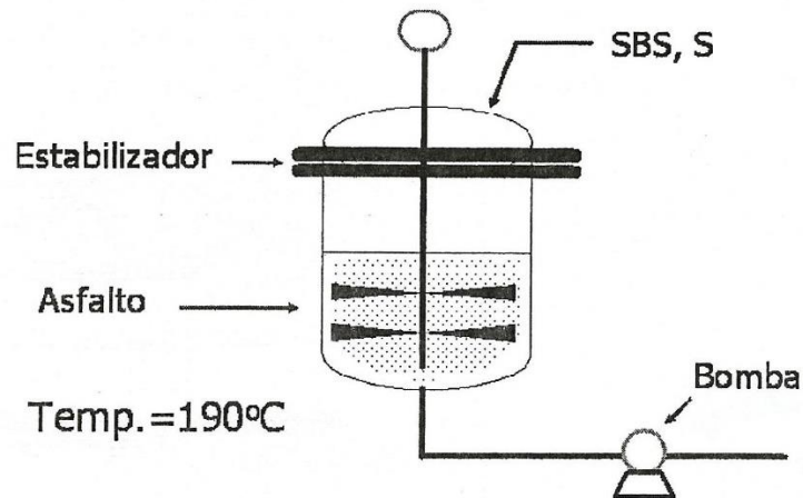
Figura 30. Diagrama de tanque de molienda cemento asfáltico – co polímero SBS
