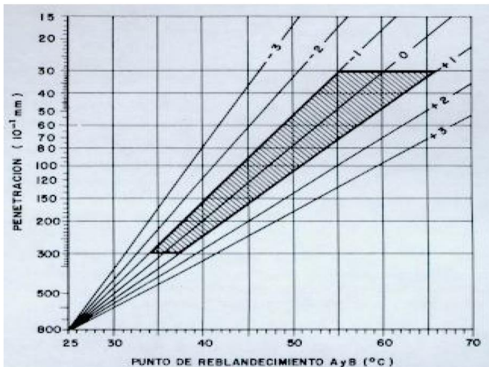
Figura 8. Índice de penetración del asfalto
