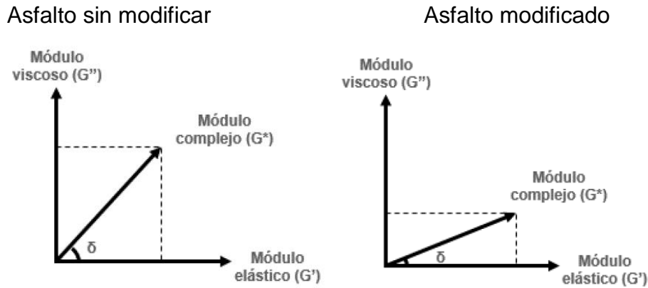
Figura 16. Módulo de corte reológico (viscosidad vs. elasticidad)
