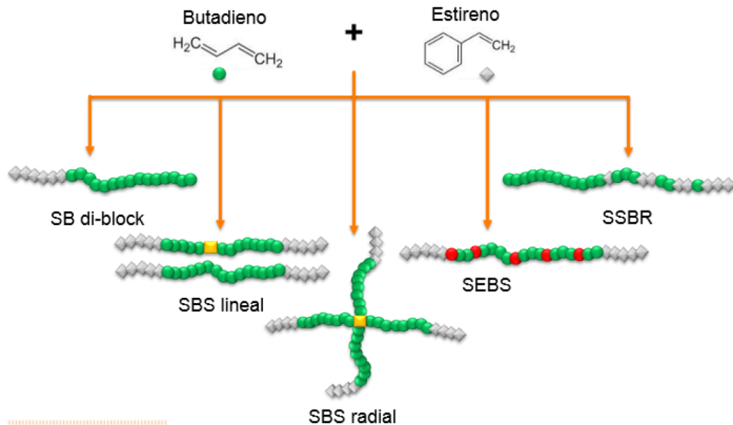
Figura 20. Co polímeros de estireno- butadieno
