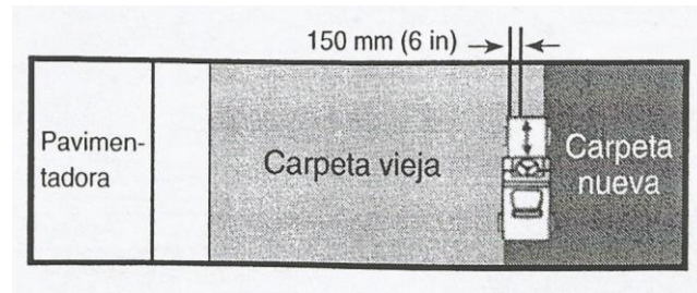
Figura 60. Compactación en junta transversal
