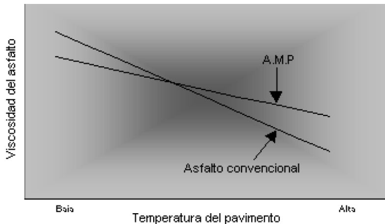
Figura 17. Efecto de un polímero sobre la rigidez y la temperatura del asfalto
