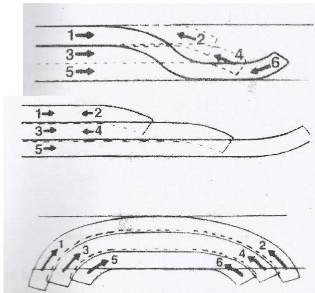
Figura 57. Patrones de compactación
