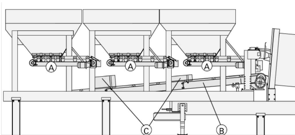
Figura 35. Vista lateral, sistema dosificador
