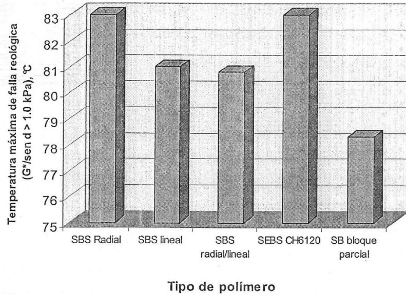
Figura 24. Temperatura máxima de falla reológica, análisis DSR
