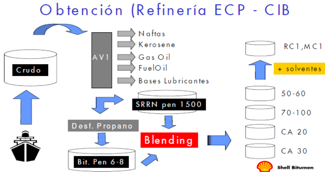
Figura 2. Proceso de refinación del petróleo
