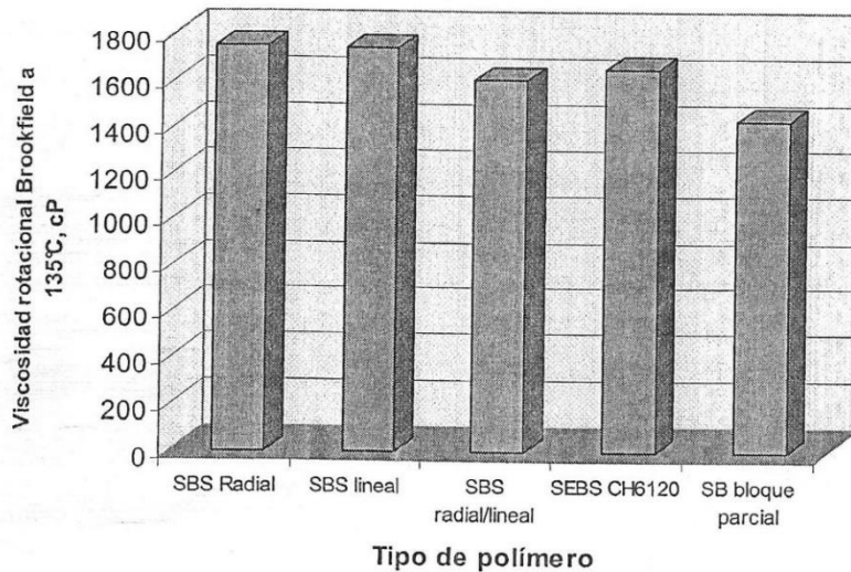
Figura 23. Viscosidad rotacional a 135°C de cemento asfáltico modificado con diferentes co polímeros de estireno-butadieno.
