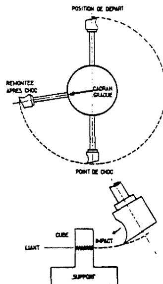
Figura 11. Mecanismo de péndulo de Vialit
