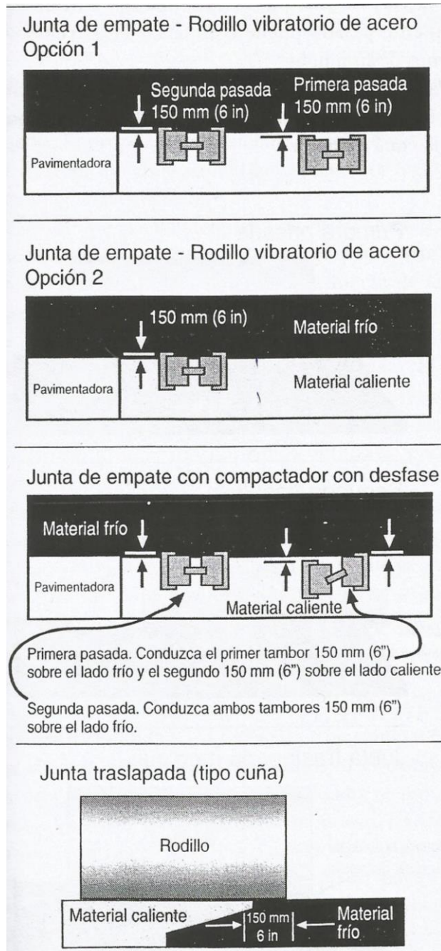
Figura 59. Compactación en junta longitudinal
