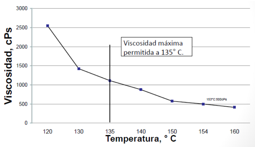
Figura 38. Viscosidad cPs vs. temperatura. manejo de asfalto en planta
