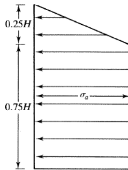
Figura 10.6 Envolverte de presión aparente para cortes en arcillas blandas y medias según Peck (1969)
