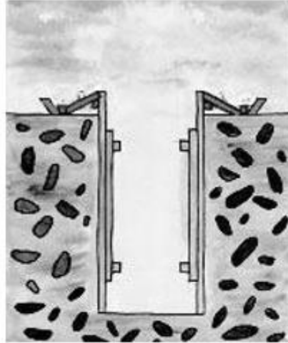
Figura 54. Sistema de anclaje de las paredes de la entibación
