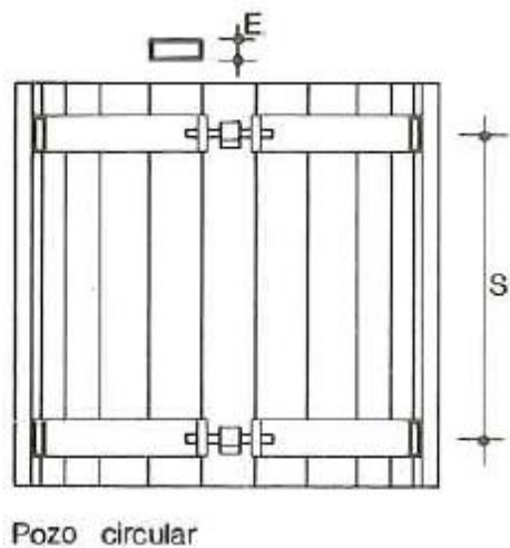
Figura 35. Simbología de entibación cuajada, aplicada a la tabla VII
