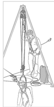
Figura 48. Sistema de ascenso y descenso, con la correcta implementación de arnés y línea de vida
