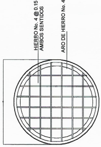
DETALLE DE TAPADERA PLANTA
