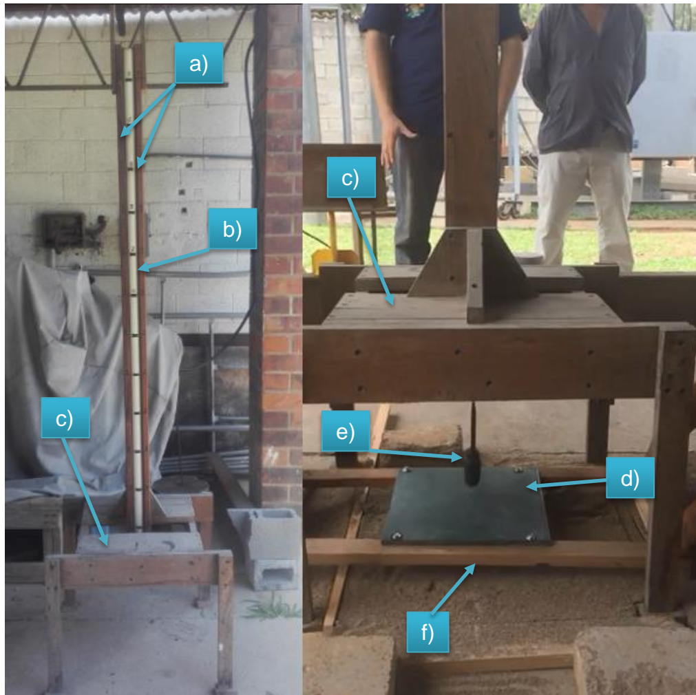
Figura 37. Equipo ensayo de impacto
