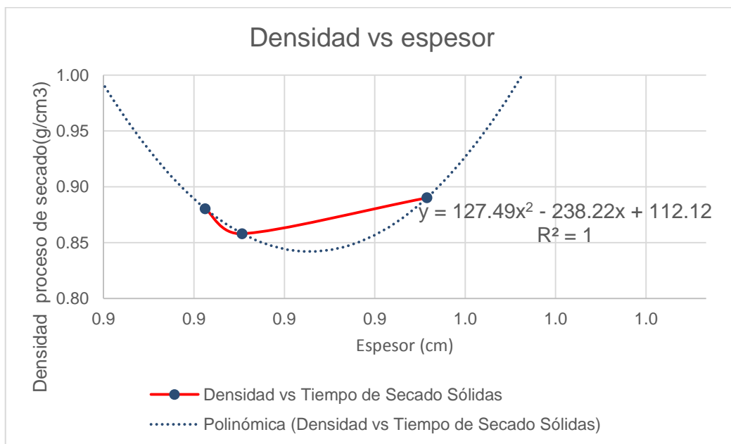
Figura 79. Densidad proceso de secado vs espesor
