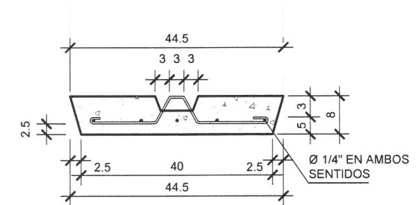
DETALLE DE TAPADERA ESCALA 1:5
