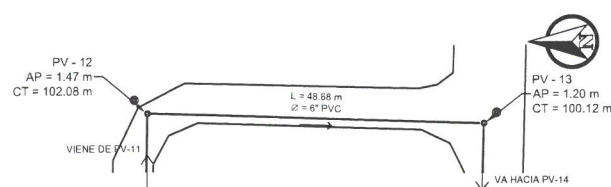
PLANTA DE PV-12 A PV-13
