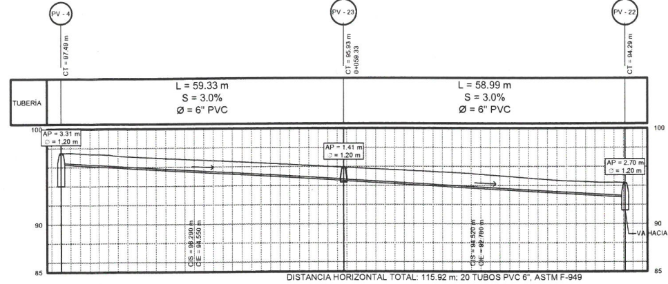
PERFIL DE PV-4 A PV-22
