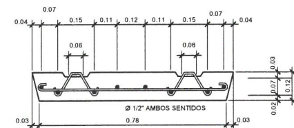
SECCIÓN C-C' TAPADERA ESCALA 1:10
