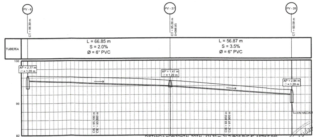
PERFIL DE PV-6 A PV-26
