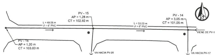
PLANTA DE PV-16 A PV-14
