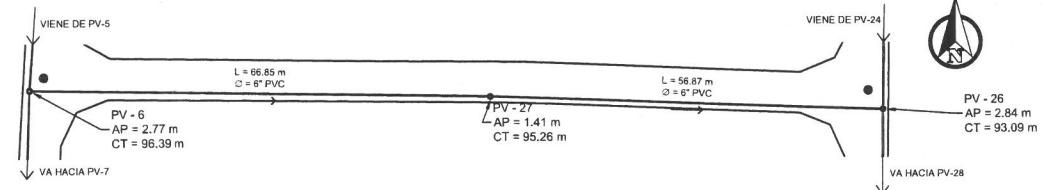
PLANTA DE PV-6 A PV-26
