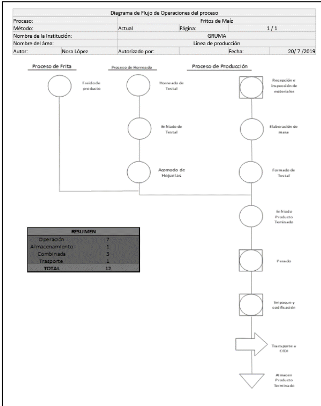
Figura 13. Diagrama de proceso
