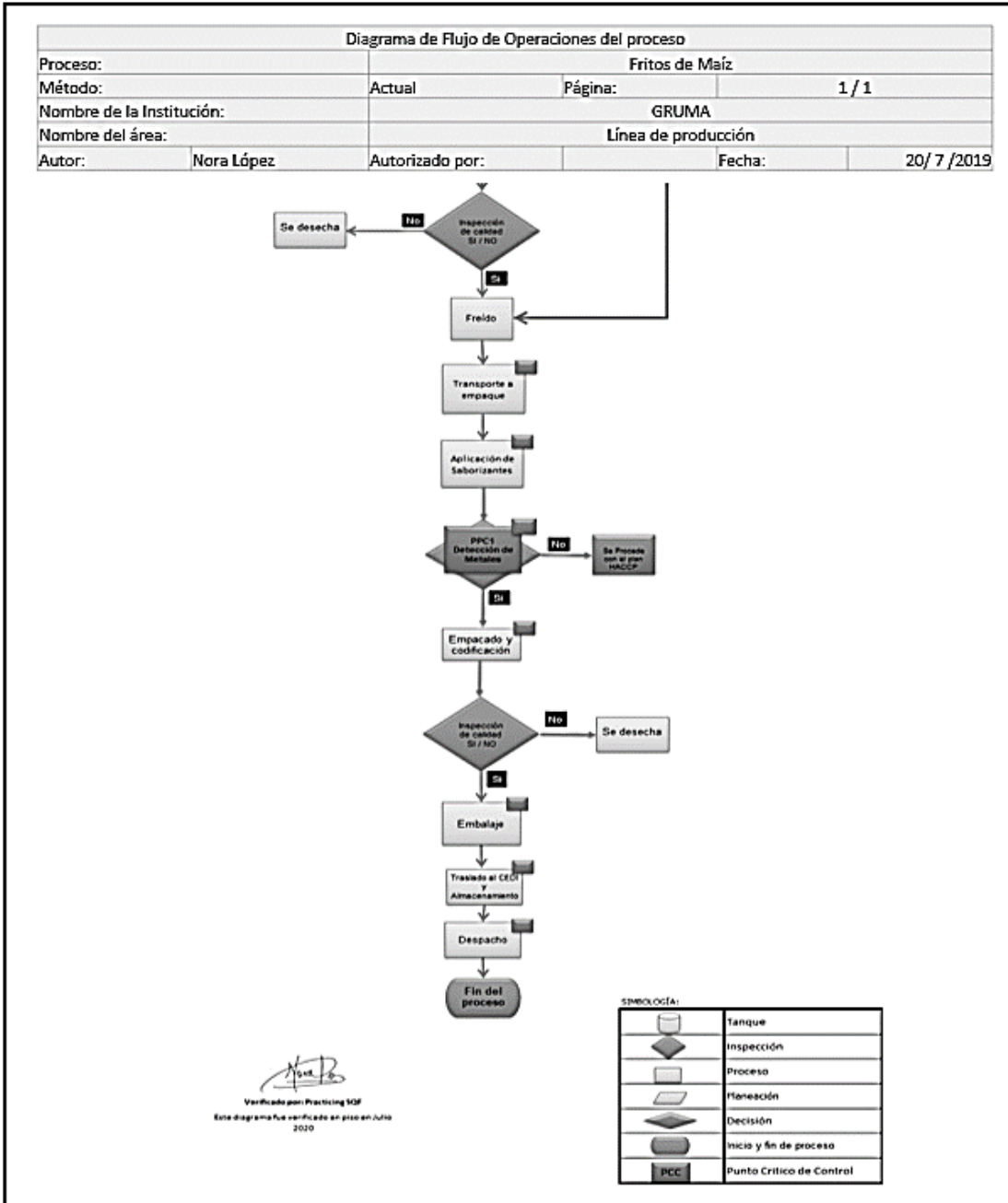
Figura 19. Diagrama de flujo 2/2
