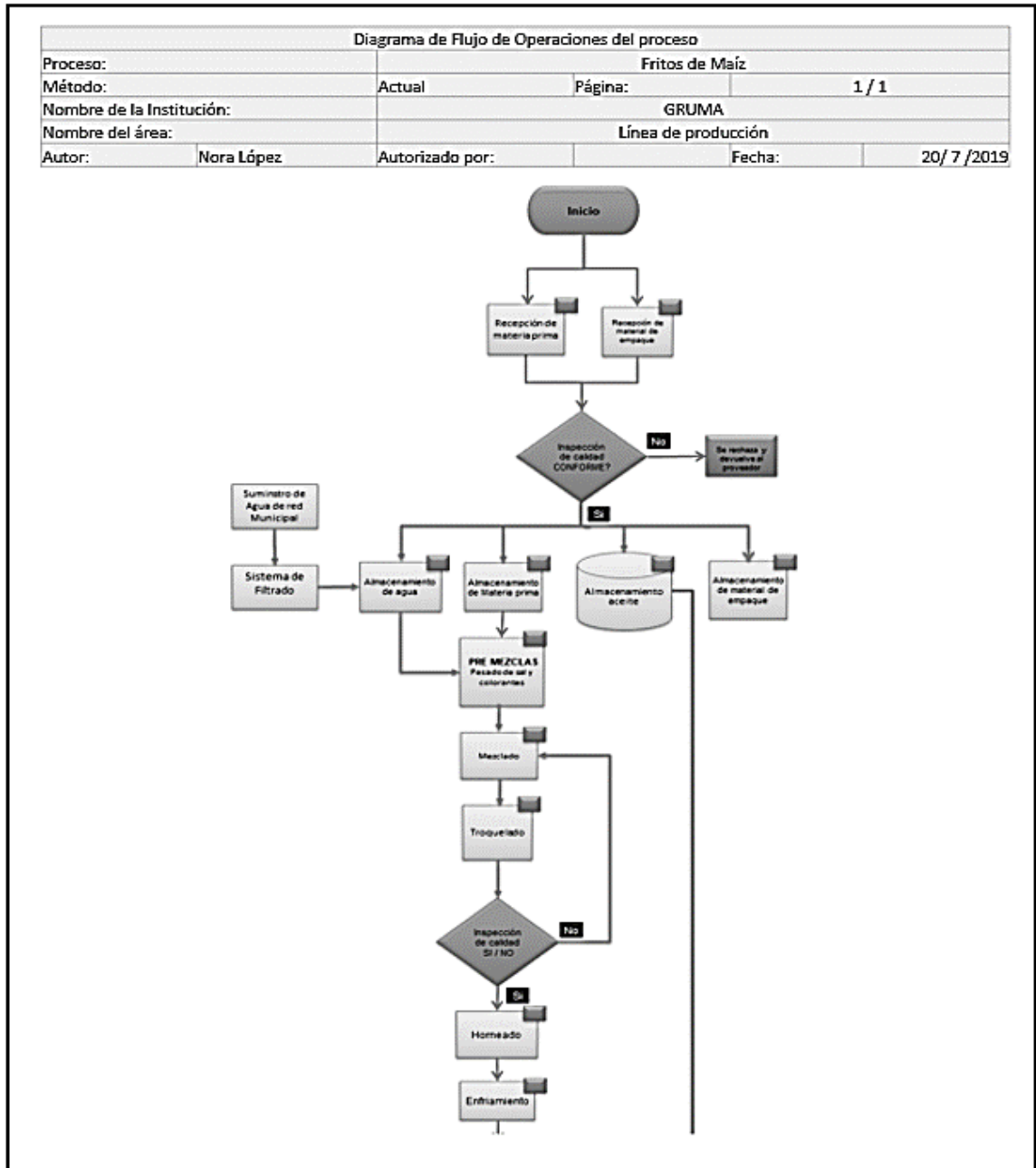
Figura 18. Diagrama de flujo 1/2
