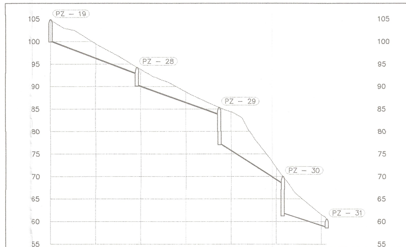
PERFIL LONGITUDINAL - PZ 19 - PZ 31
