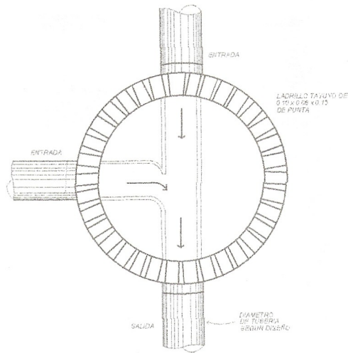
PLANTA POZO DE VISITA DOBLE ENTRADA
