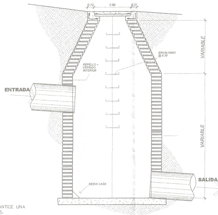
CORTE A-A'
