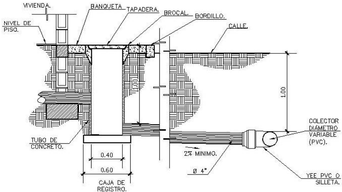
Figura 8. Detalle conexiones domiciliarias
