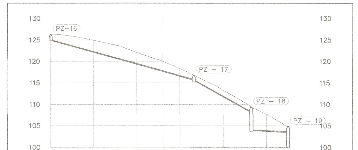
PERFIL LONGITUDINAL - PZ 16 - PZ 19
