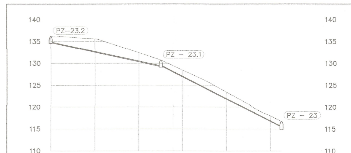
PERFIL LONGITUDINAL - PZ 23.2 - PZ 23
