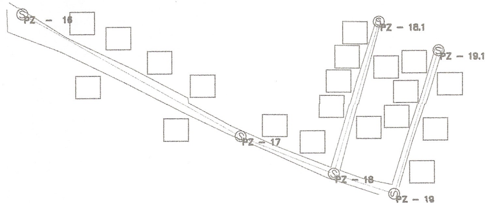
PLANTA PZ 16 - PZ 19
