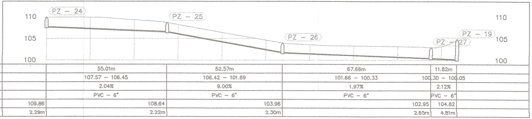
PERFIL PZ 19 - PZ 24
