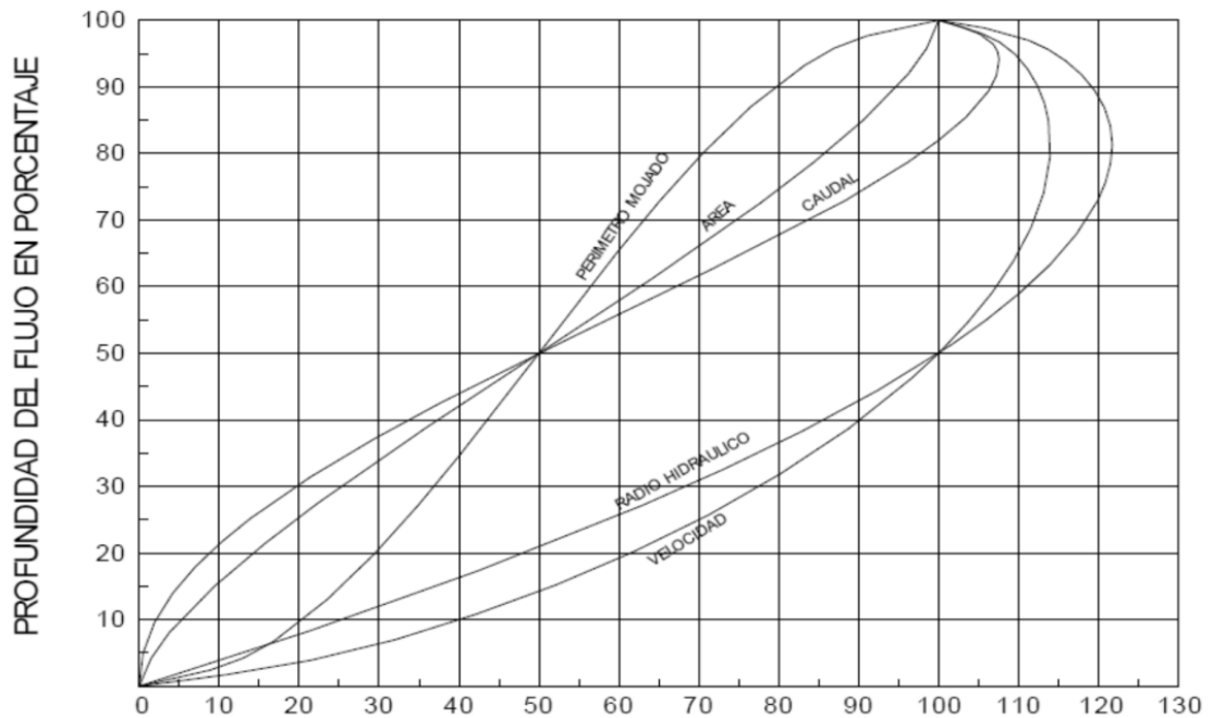
Figura 10. Diagrama de relaciones hidráulicas de una tubería de sección circular parcialmente llena
