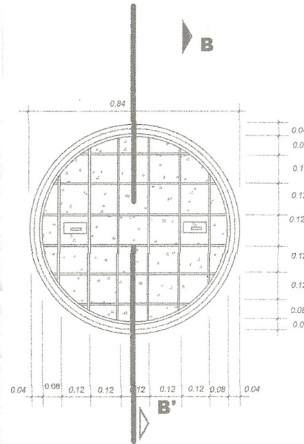
DETALLE DE ARMADO
