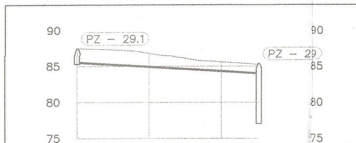
PERFIL LONGITUDINAL - PZ 29.1 - PZ 29
