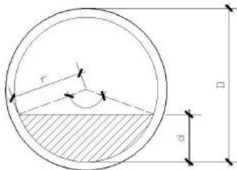
Figura 9. Sección transversal de tubería
