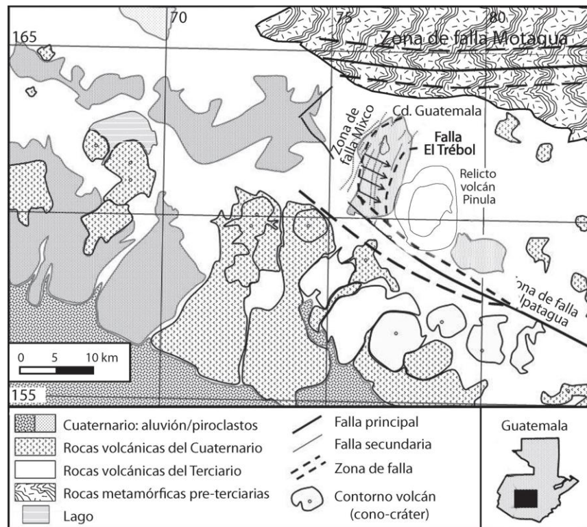
Figura 4. Modelo tectónico que interpreta la estructura del Valle de Guatemala
