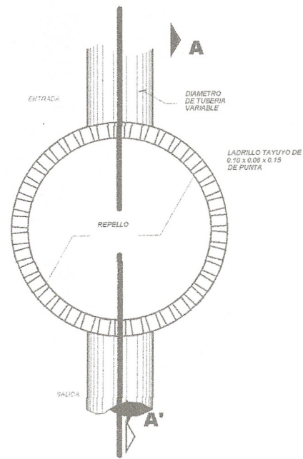
PLANTA POZO DE VISITA UNA ENTRADA
