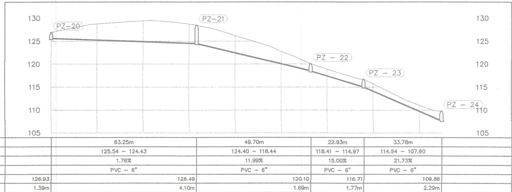
PERFIL PZ 23.2 - PZ 23
