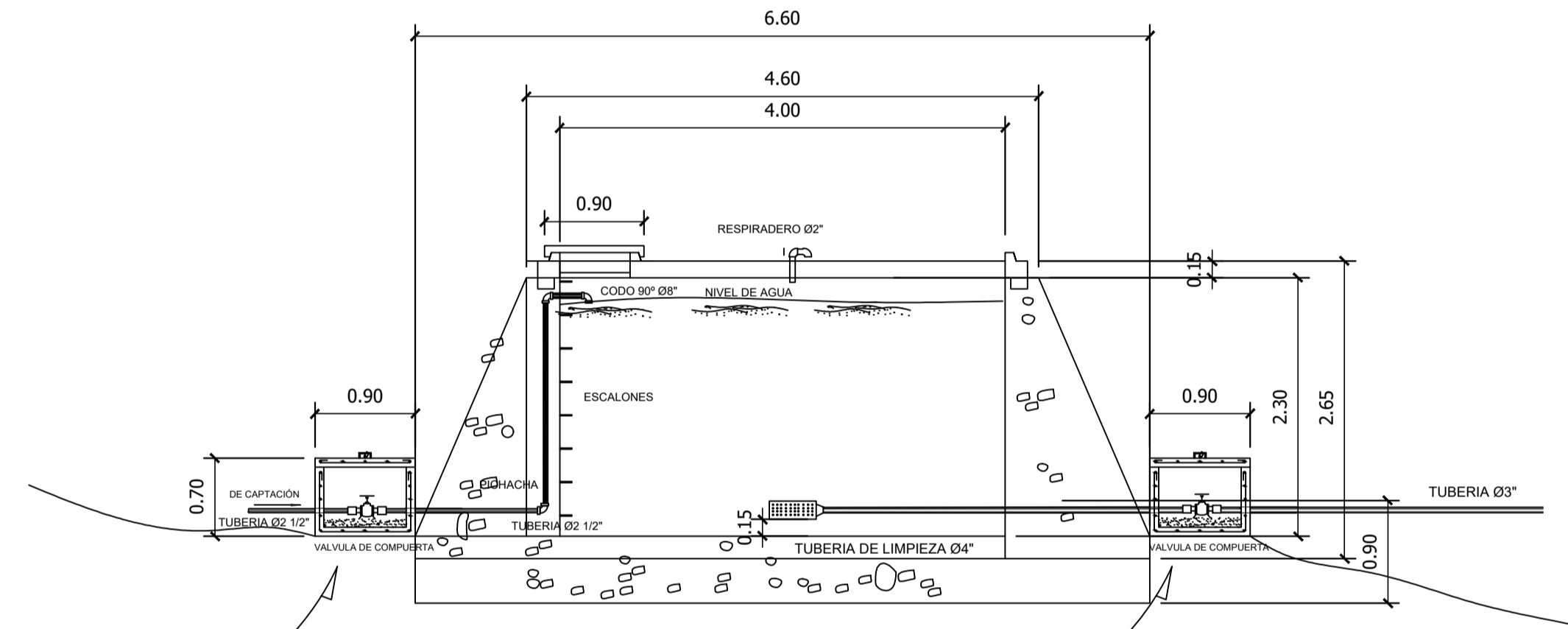
SECCION "B" TANQUE DE ALMACENAMIENTO ESCALA 1:100
