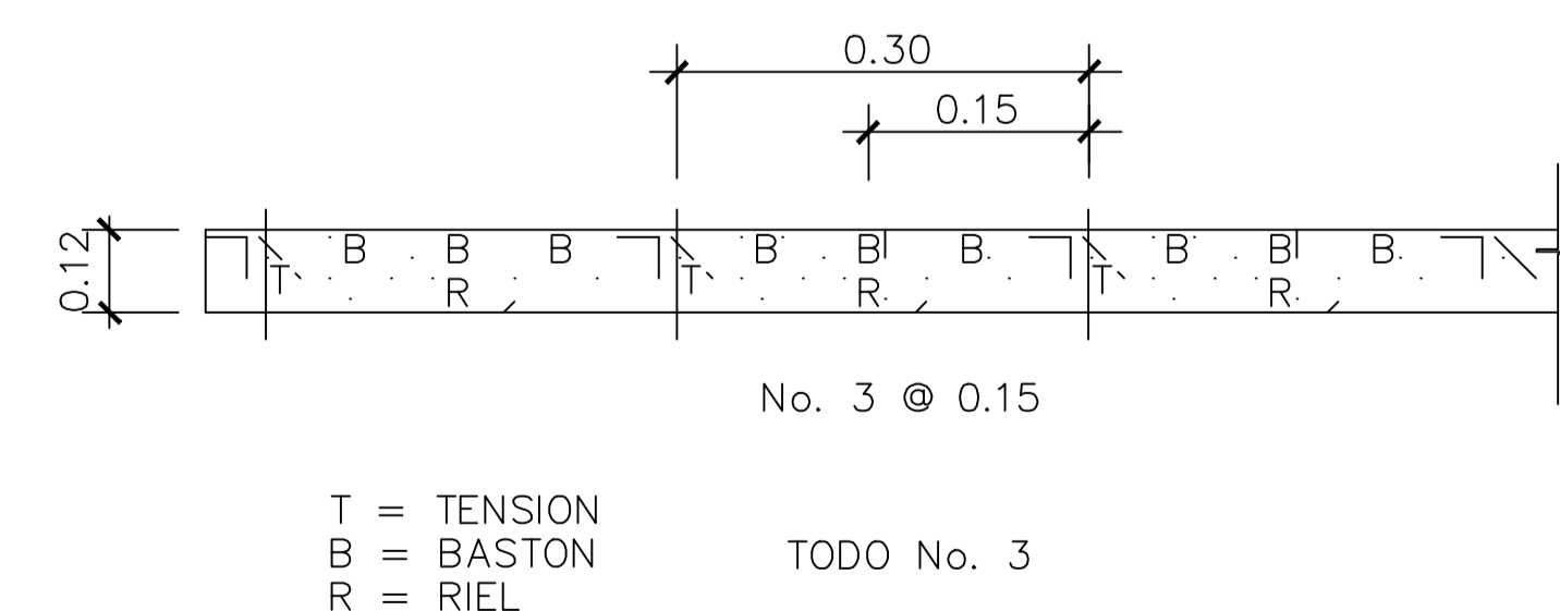
DETALLE DE ARMADO DE LOSA ESCALA 1:100
