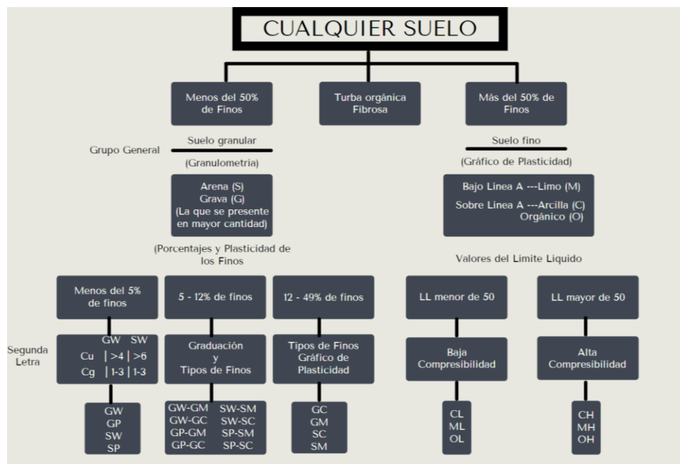
Figura 39. Diagrama de clasificación SUCS
