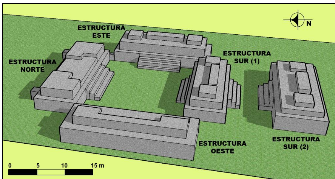
Figura 21. Reconstrucción digital del Grupo 25. (Dibujo de Claudia Valenzuela)
