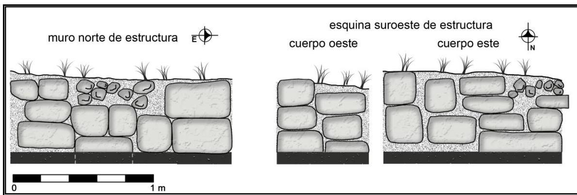
Figura 27. Cortes de muros de estructura sobre piso estucado que marca la nivelación artificial del grupo. (Dibujo de Claudia Valenzuela)
