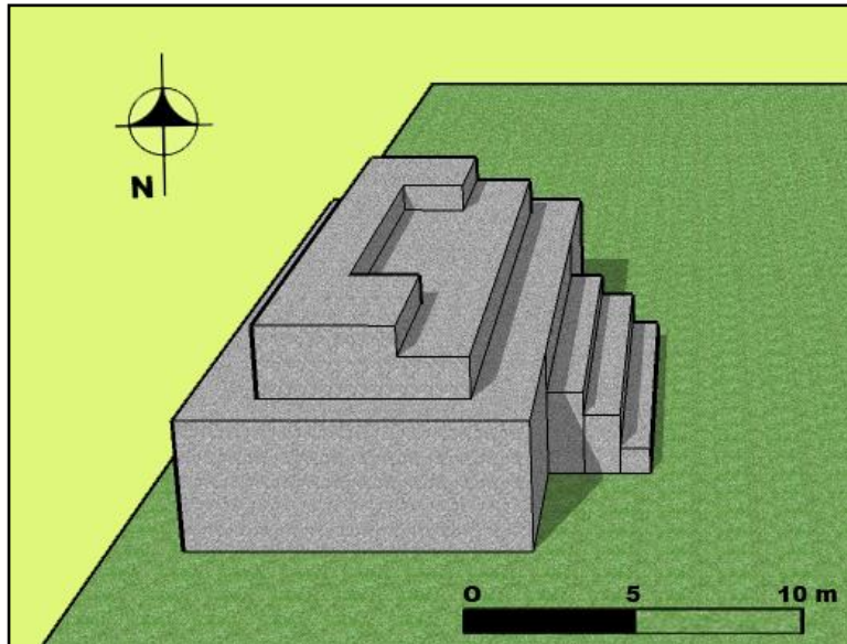
Figura 33. Reconstrucción digital de estructura oeste, mostrando su banqueta superior en forma de “C”.(Dibujo de Claudia Valenzuela)
