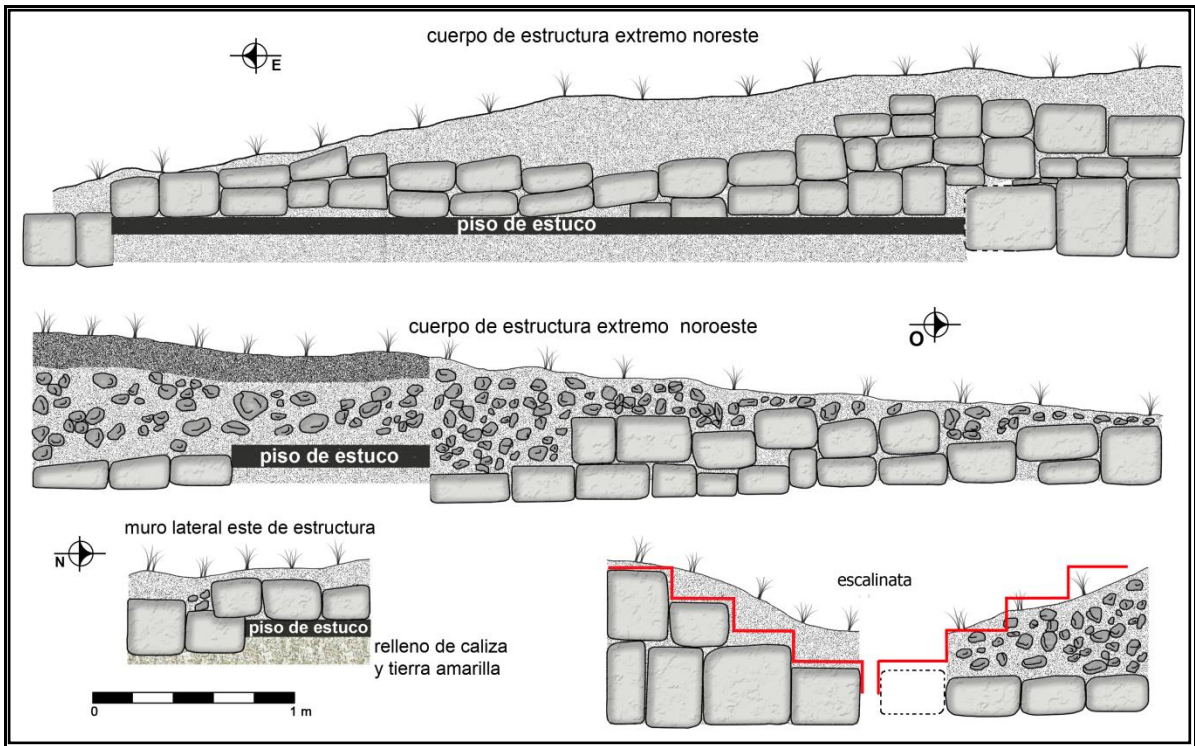
Figura 30. Cuerpo frontal de estructura Sur 25-3 (1), mostrando la nivelación del piso de estuco dentro de la plaza. (Dibujo de Claudia Valenzuela)
