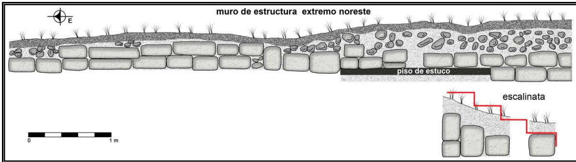
Figura 32. Muro frontal de Estructura Sur 25-2. (Dibujo de Claudia Valenzuela)
