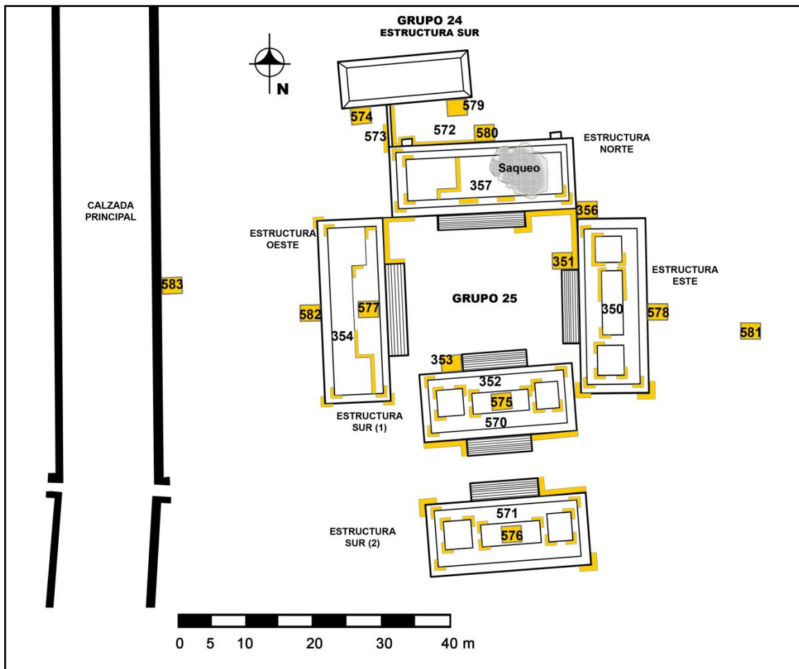
Figura 40. Mapa del Grupo 25 con las unidades de excavación realizadas. (Dibujo de Claudia Valenzuela)
