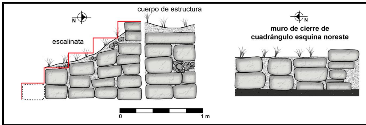
Figura 22. Lateral de escalinata y muro frontal de estructura. (Dibujo de Claudia Valenzuela)
