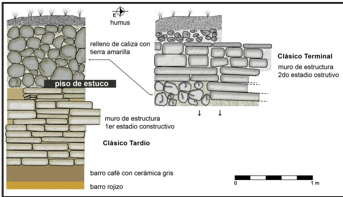
Figura 39. Cortes norte de estructura sur de Grupo 24, marcando la estratigrafía cultural del área sur de Pueblito. (Dibujo de Claudia Valenzuela)
