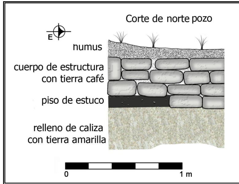
Figura 36. Corte norte de operación 351, mostrando los distintos niveles culturales que conforman el Grupo 25. (Dibujo de Claudia Valenzuela)
