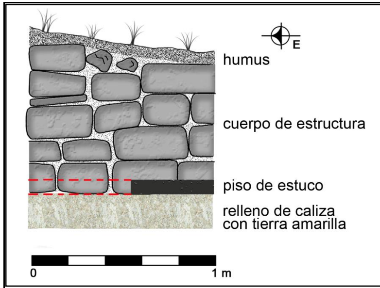
Figura 38. Corte sur de pozo donde se muestra la estratigrafía cultural dentro de la plaza del Grupo 25. (Dibujo de Claudia Valenzuela)
