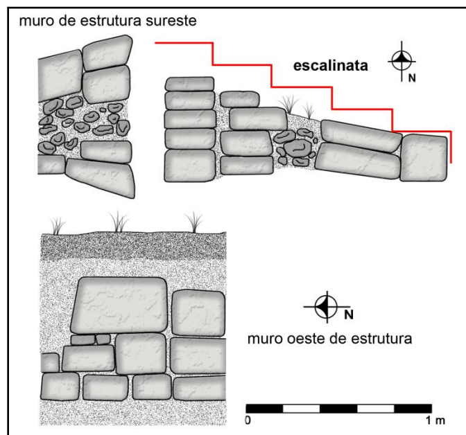
Figura 34. Muro y escalinata de estructura oeste 25-4. (Dibujo de Claudia Valenzuela)
