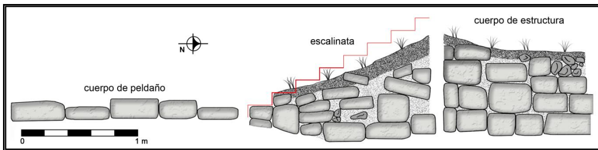
Figura 26. Escalinata y muro de estructura. (Dibujo de Claudia Valenzuela)
