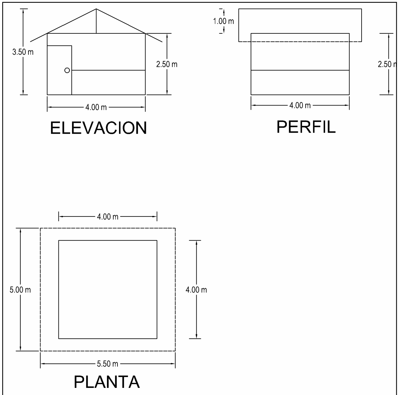
Figura 11.6. Dimensiones de la caseta de bombeo.
