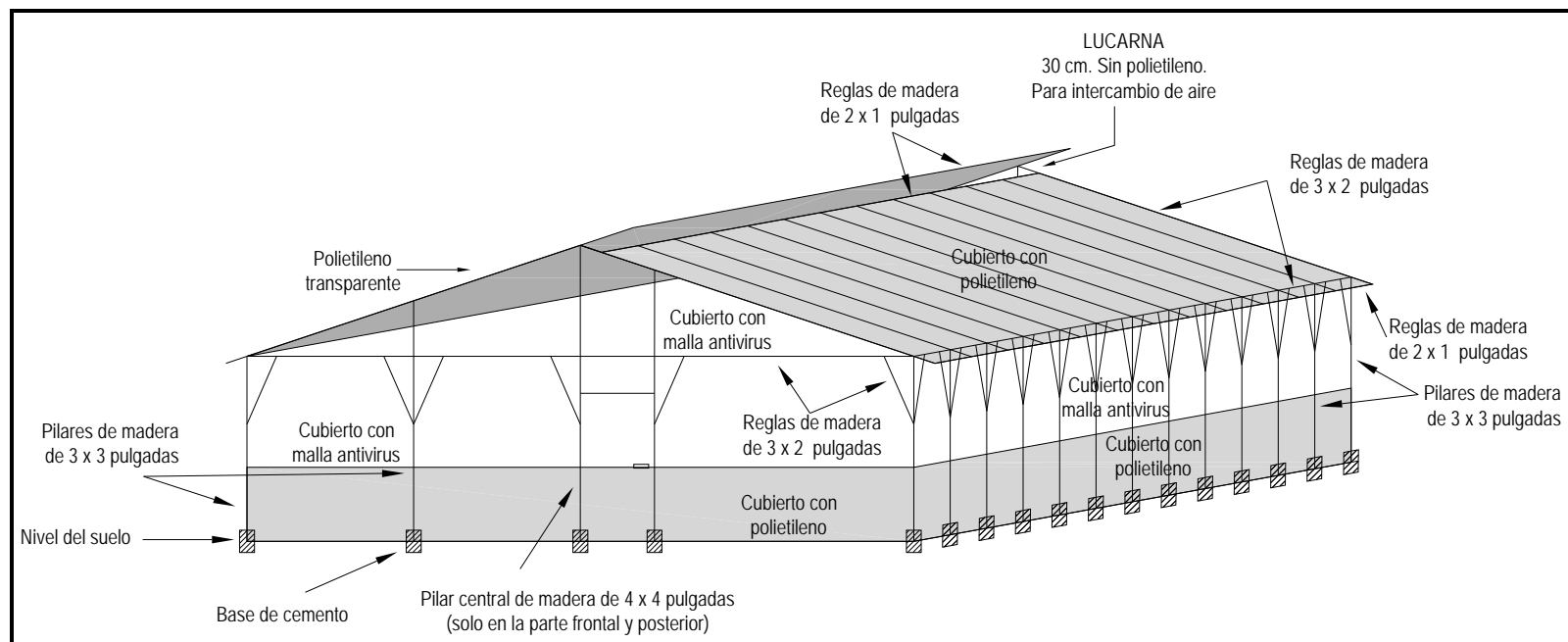
Figura 11.1. Estructura y cubierta del invernadero.
