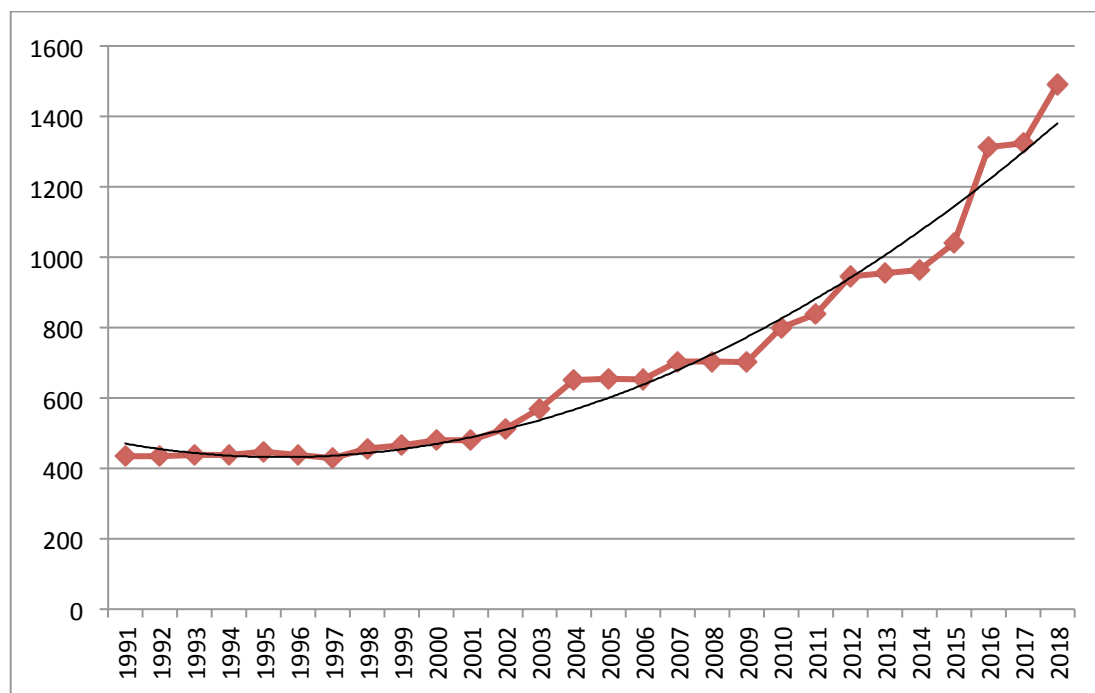
Gráfica No. 38 Capacidad instalada para producir energía eléctrica por fuente Hidroeléctrica 1991-2018 (En megavatios)
