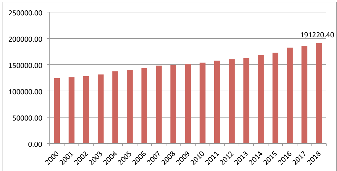
Gráfica No. 19. Capacidad instalada en hidroeléctricas para producir energía eléctrica América Latina y el Caribe 2000-2018 (En megavatios)
