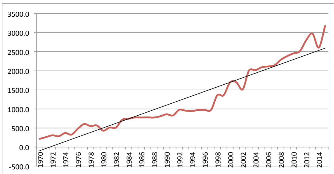
Gráfica No. 37 Capacidad instalada para producir energía eléctrica en Guatemala 1970-2015 (En megavatios)
