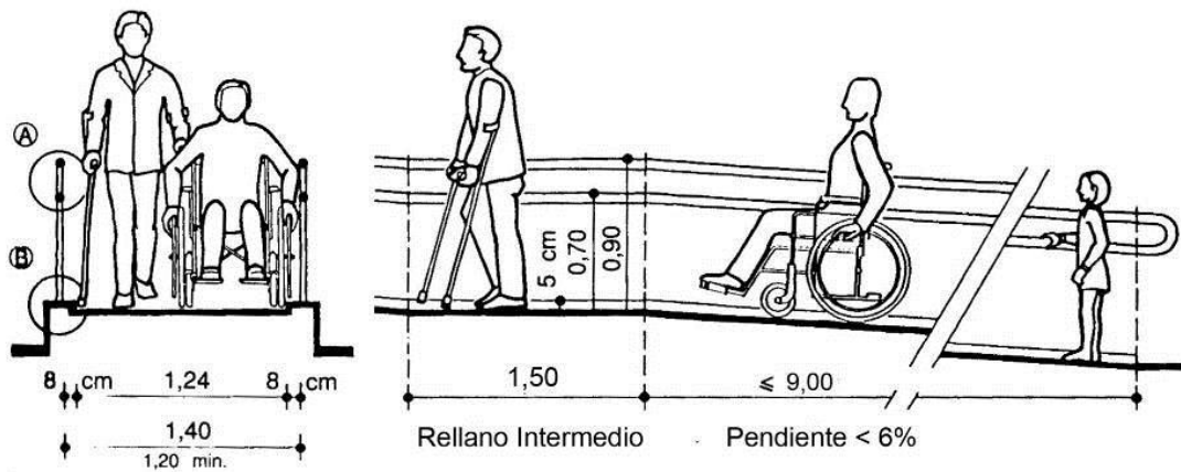
Diseño de rampa universal
