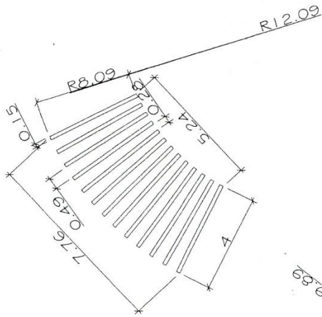
DETALLE PERGOLA 6
