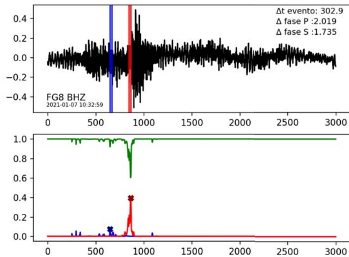
Figura 3.9. Muestra en la que no se tuvo coincidencia para ninguna de las fases sísmicas. En la parte superior aparece el sismograma de la muestra, en azul se aprecian las picadas de fase P(etiqueta y predicción) y en rojo las picadas de fase S . En la parte de abajo se ven las distribuciones de probabilidad resultantes de SeismicNet, el punto máximo que se aprecia en la gráfica marcado con una X de las distribuciones de probabilidad sirve para identificar el arribo de fase correspondiente, es decir generar una predicción. En la parte inferior izquierda del sismograma se identifica el código de la estación sísmica y el canal de la muestra, abajo aparece la hora del evento sísmico.
